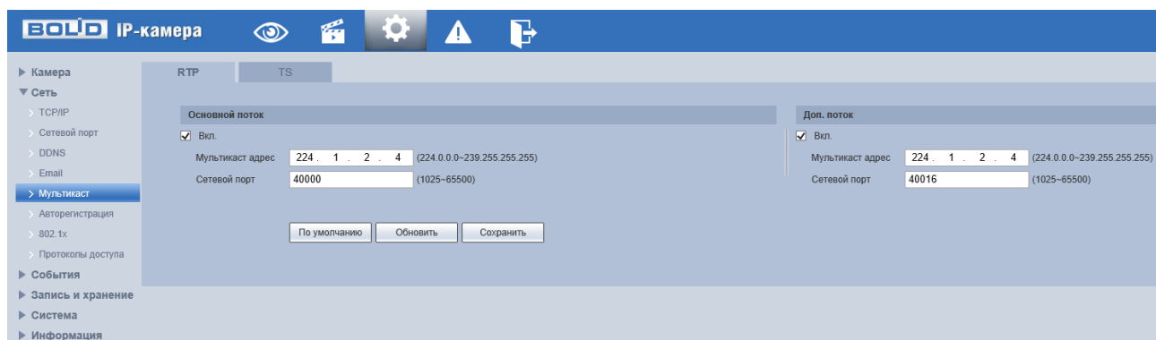
Рисунок 7.58 – Подпункт меню «Мультикаст»
