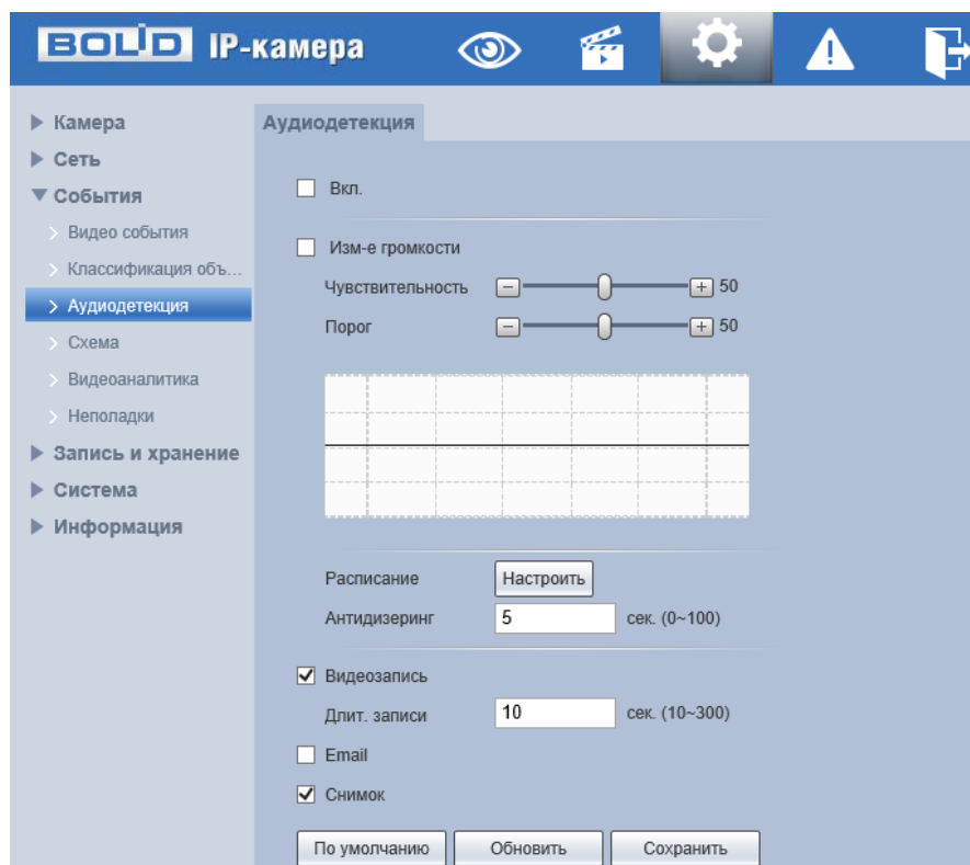
Рисунок 7.74 – Подпункт меню «Аудиодетекция»
