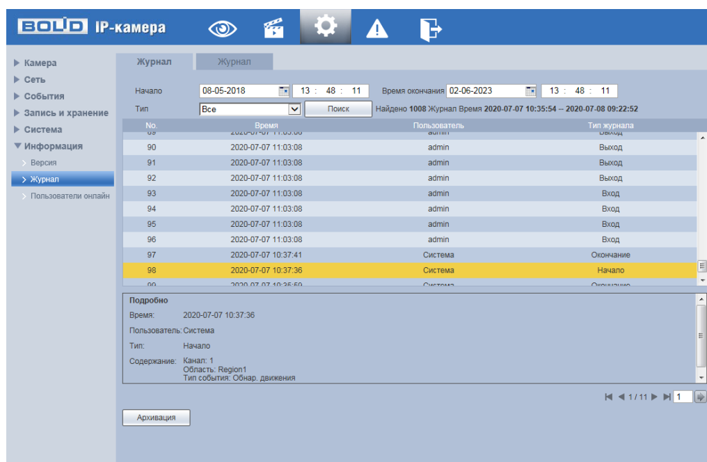
Рисунок 7.122 – Просмотр подробной информации о системном событии
