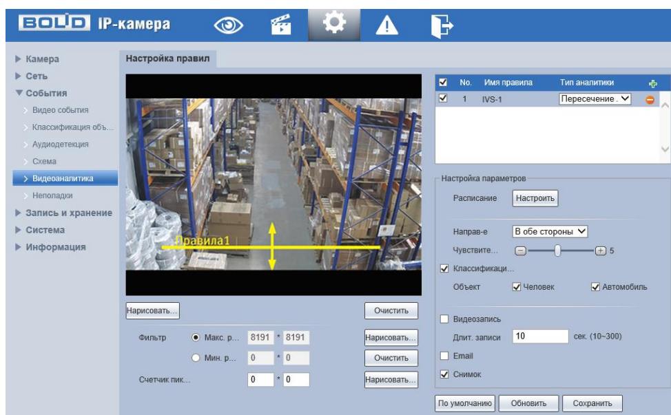
Рисунок 7.77 – Создание правила видеоаналитики «Пересечение линии»
