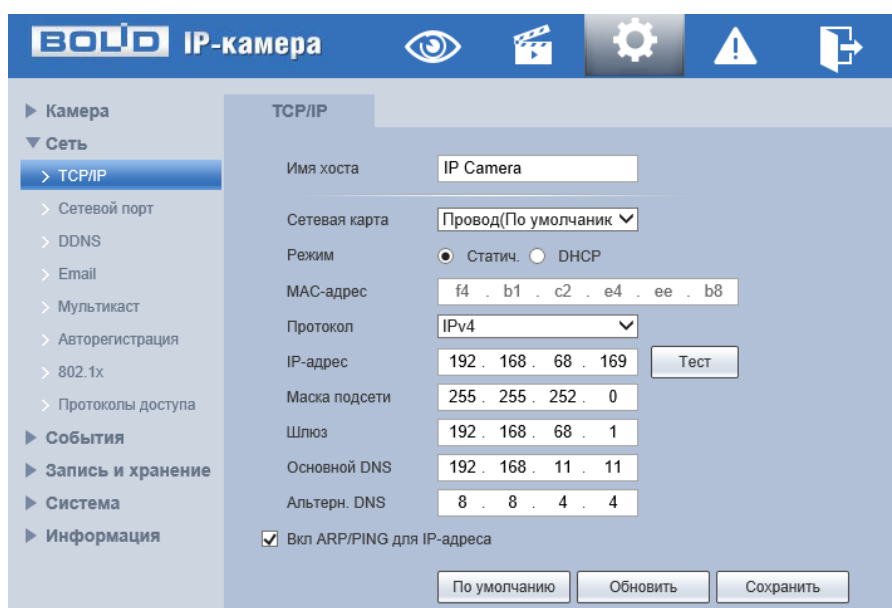
Рисунок 7.52 – Подпункт меню «TCP/IP»
