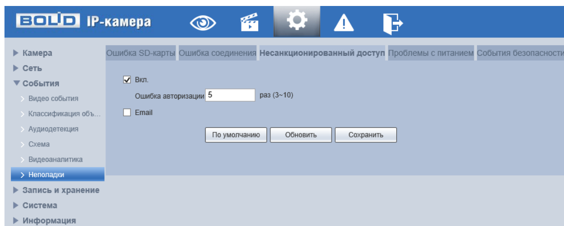
Рисунок 7.82 – Вкладка «Несанкционированный доступ»
