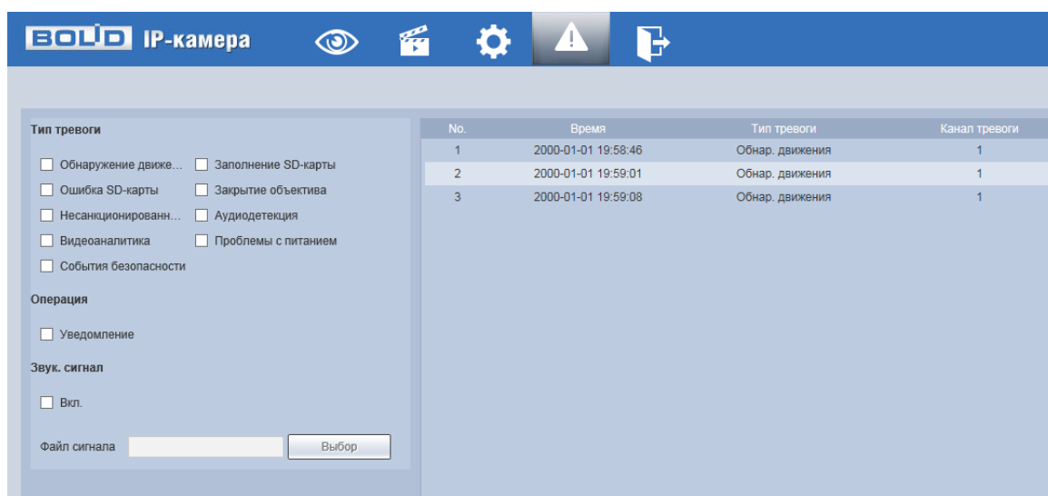
Рисунок 7.125 – Раздел меню «События»
