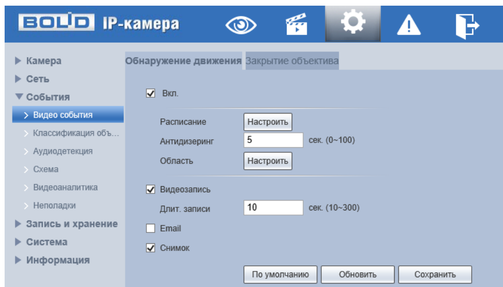
Рисунок 7.68 – Вкладка «Обнаружение движения»
