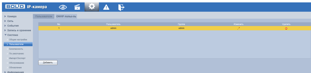
Рисунок 7.105 – Вкладка «ONVIF пользователь»
