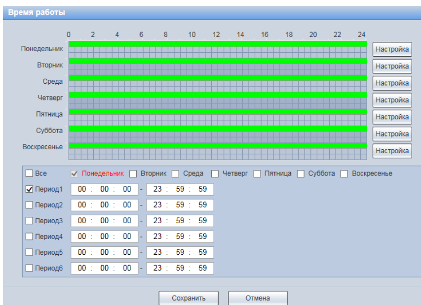
Рисунок 7.69 – Вкладка «Обнаружение движения»: Расписание
