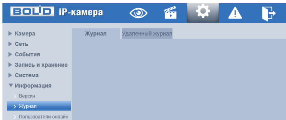
Рисунок 7.120 – Подпункт меню «Журнал»
