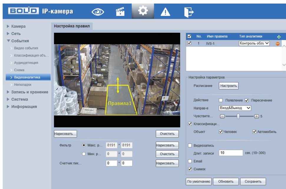
Рисунок 7.78 – Создание правила видеоаналитики «Контроль области»
