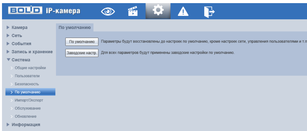
Рисунок 7.112 – Подпункт меню «По умолчанию»
