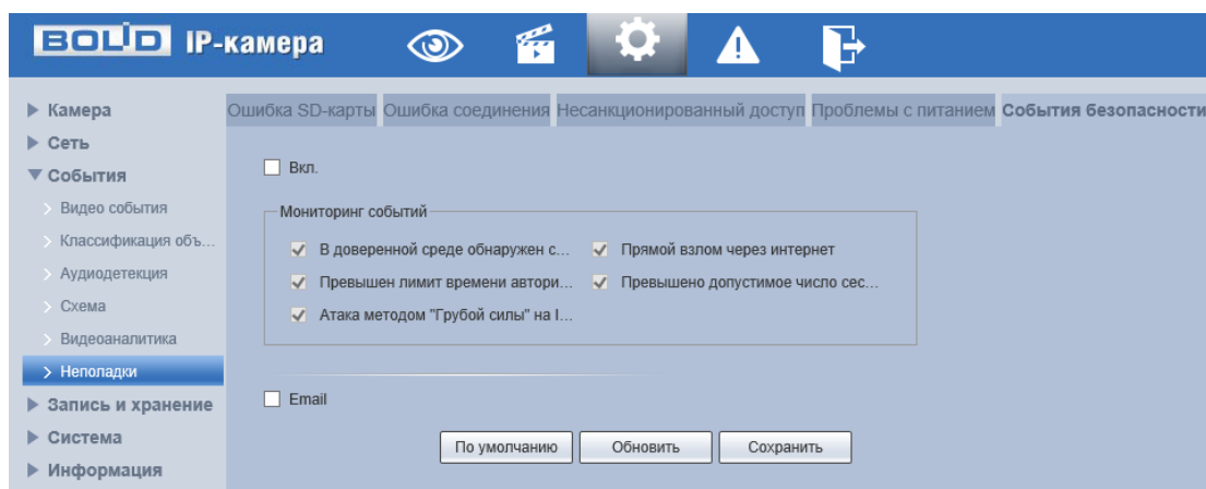
Рисунок 7.84 – Вкладка «События безопасности»
