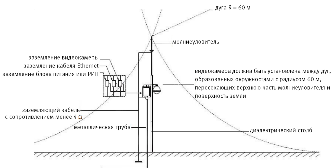
Рисунок 6.12 – Установка молниеотвода
