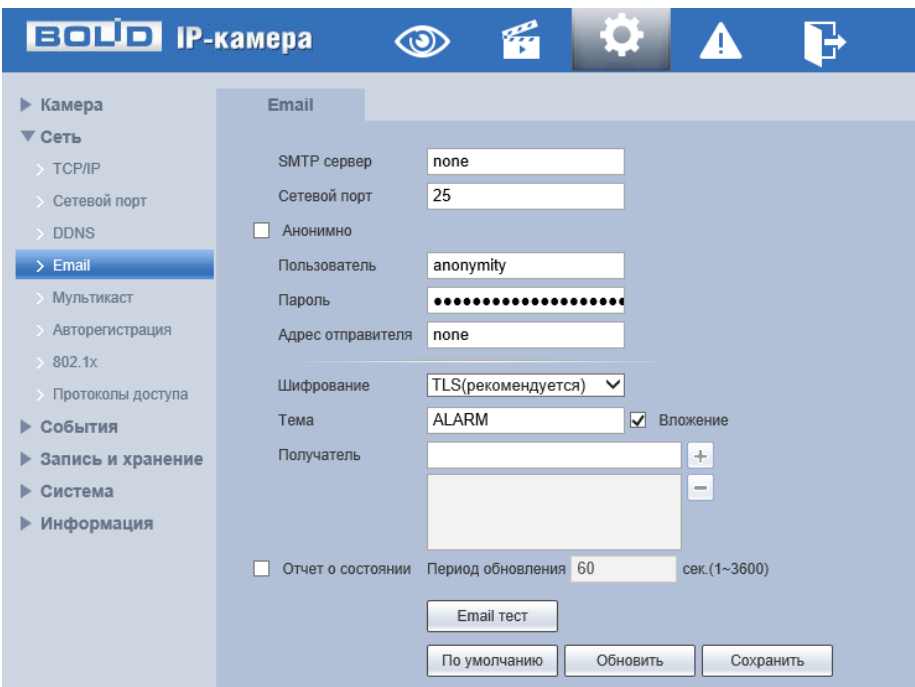
Рисунок 7.56 – Подпункт меню «Email»
