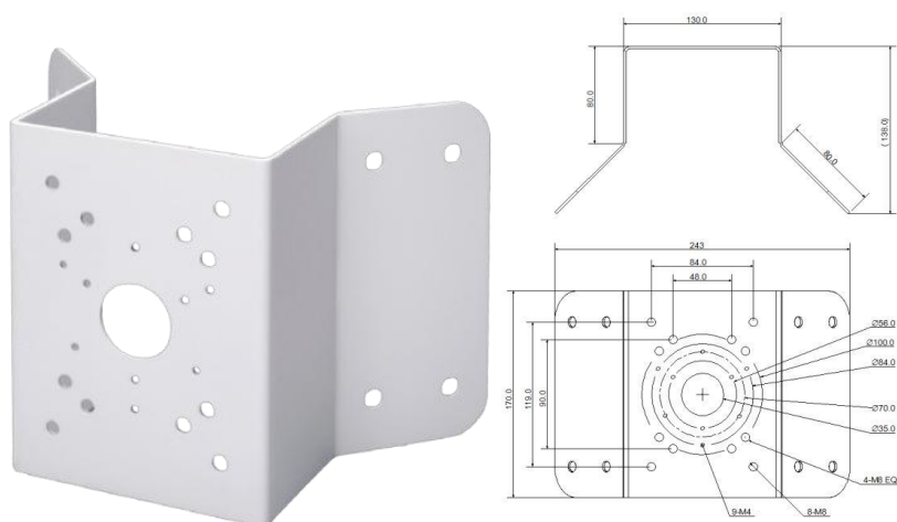
Рисунок 5.10 – Угловой кронштейн BR-102
