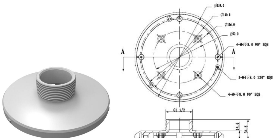
Рисунок 5.5 – Монтажный адаптер BR-303
