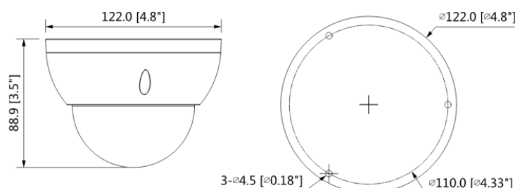
Рисунок 5.1 – Габаритные размеры видеокамеры
