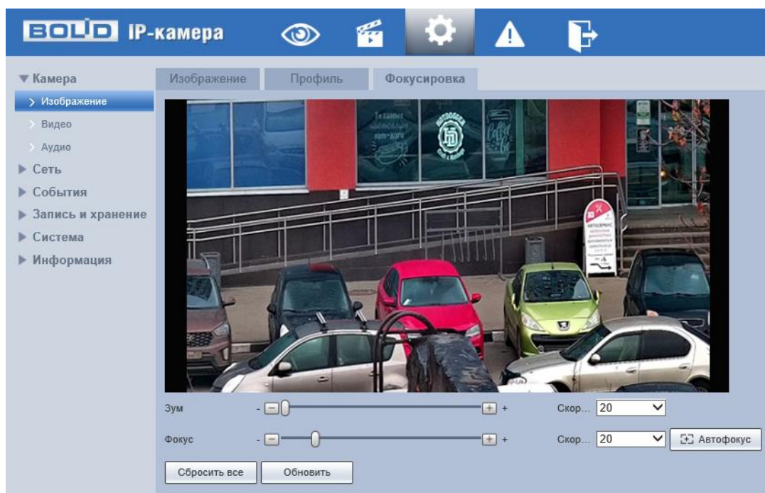
Рисунок 7.39 – Вкладка «Фокусировка»
