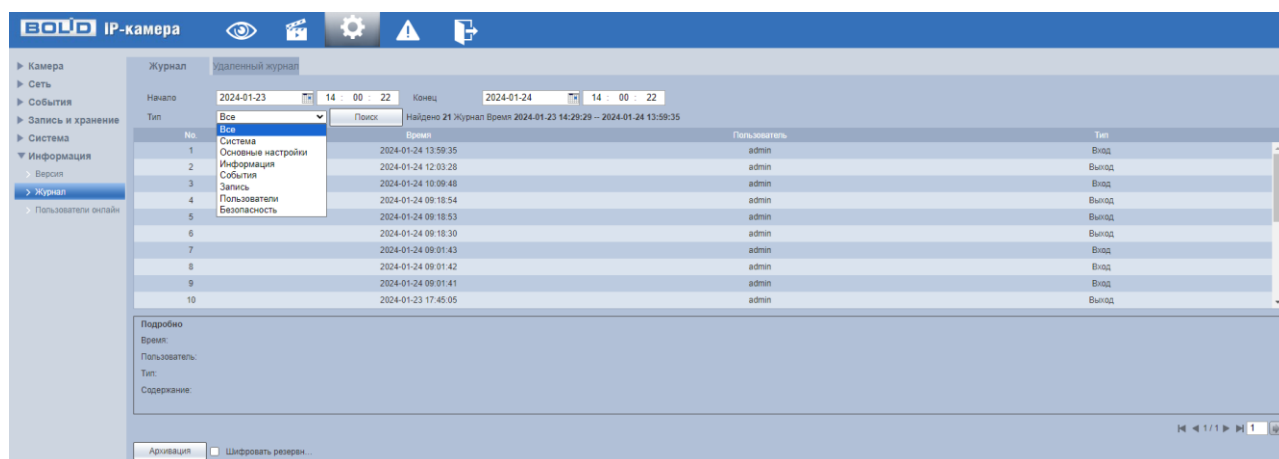
Рисунок 7.129 – Вкладка «Журнал»
