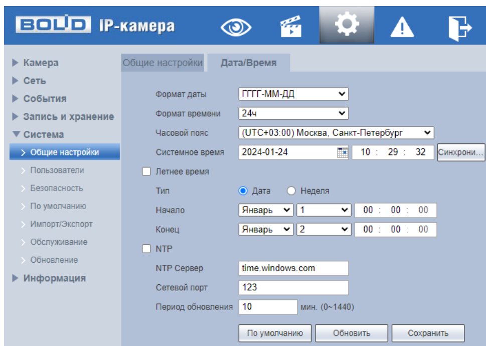
Рисунок 7.105 – Вкладка «Дата/Время»
