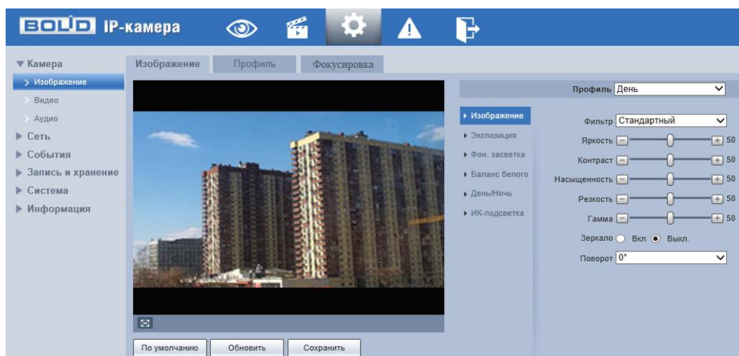
Рисунок 7.29 – Вкладка «Изображение»
