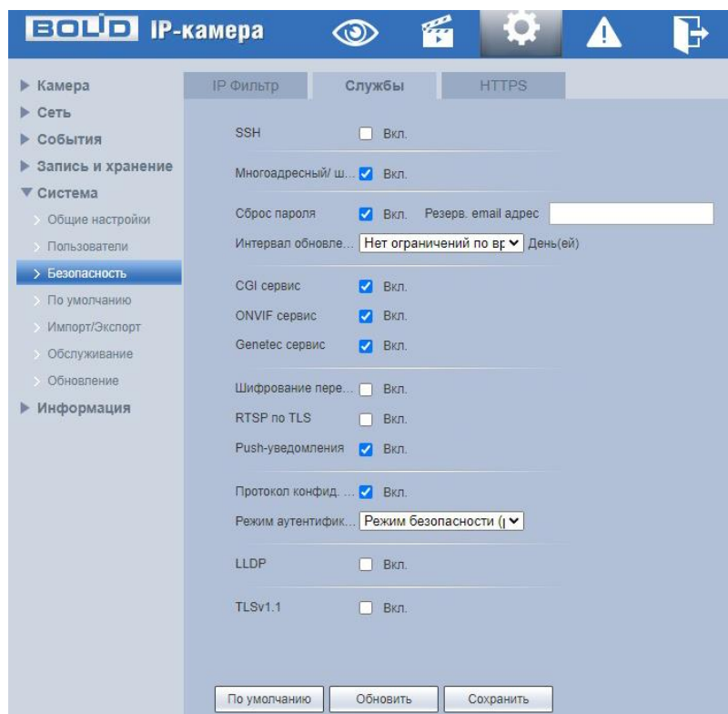
Рисунок 7.117 – Вкладка «Службы»
