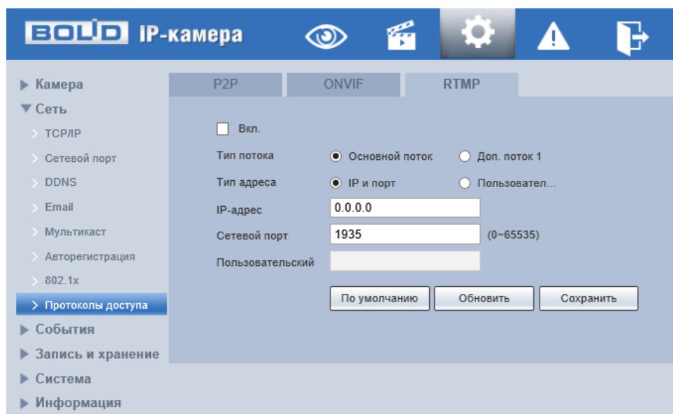
Рисунок 7.66 – Вкладка «RTMP»
