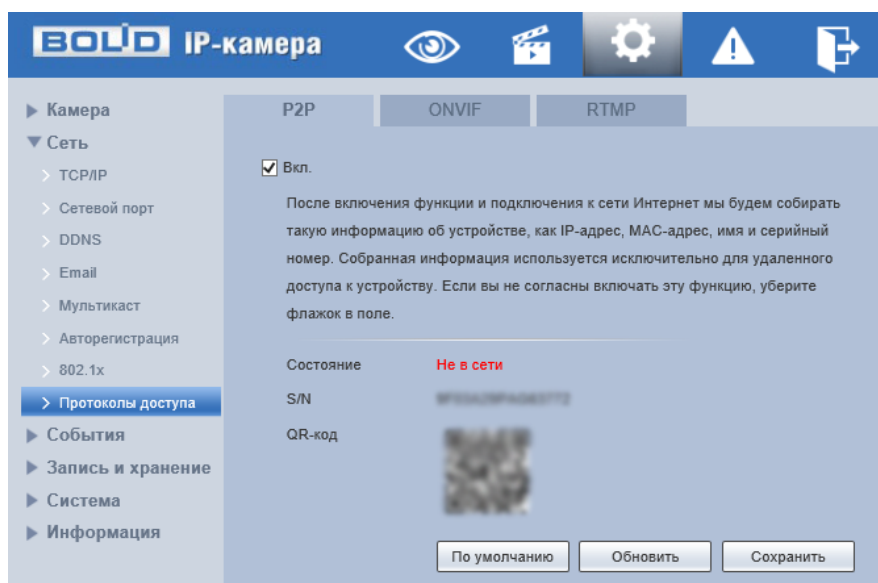
Рисунок 7.64 – Вкладка «P2P»
