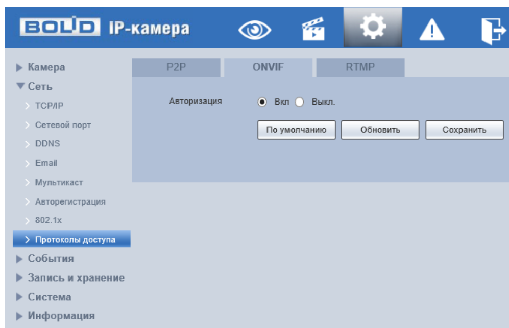
Рисунок 7.65 – Вкладка «ONVIF»
