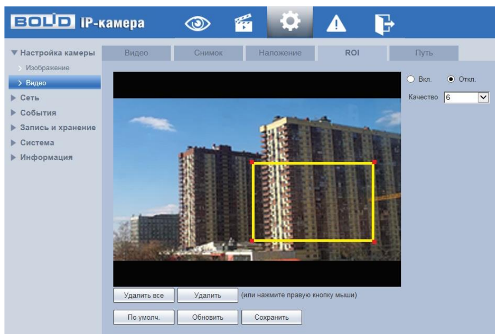
Рисунок 7.49 – Вкладка «ROI»
