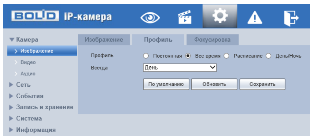
Рисунок 7.38 – Вкладка «Профиль»
