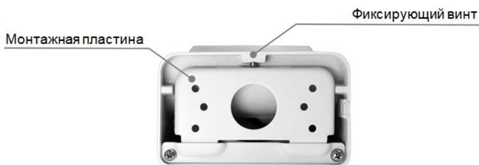
Рисунок 5.5 – Настенный кронштейн
