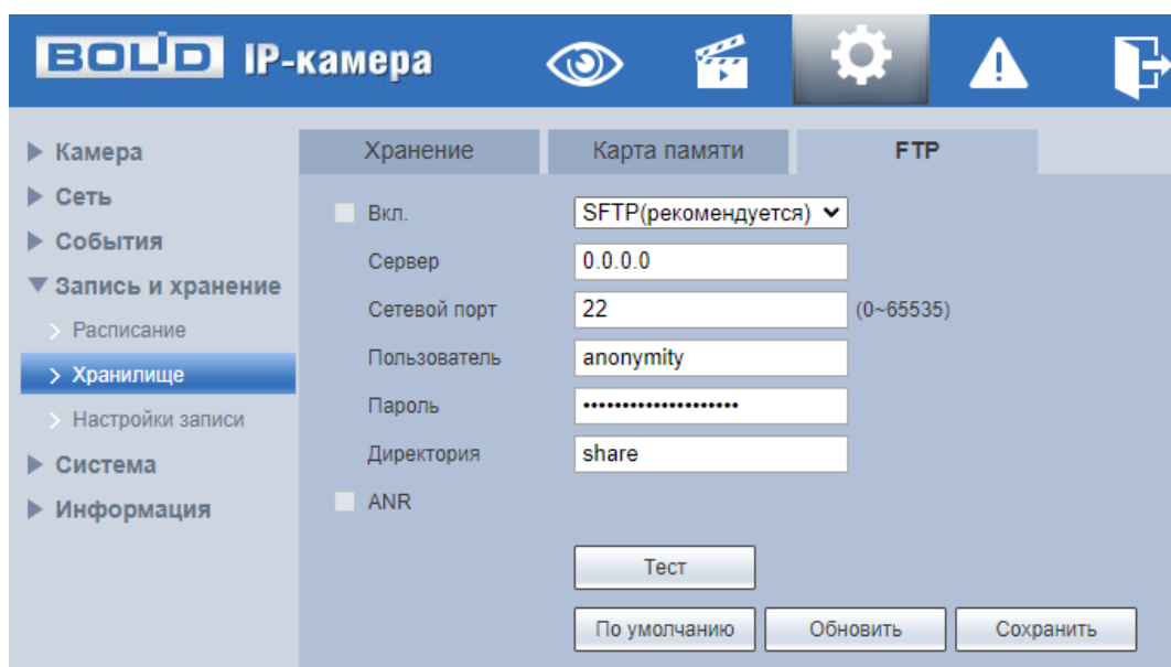
Рисунок 7.96 – Вкладка «FTP»
