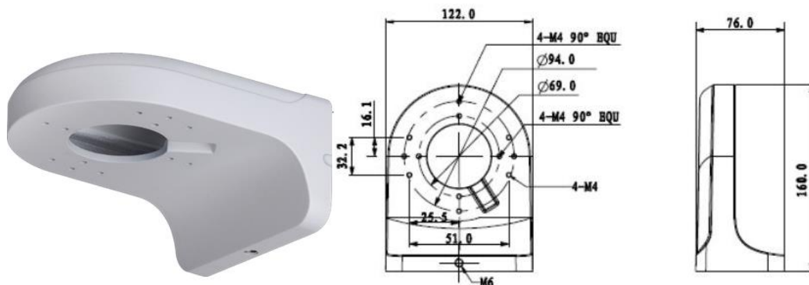
Рисунок 5.4 – Внешний вид и габаритные размеры кронштейна BR-106
