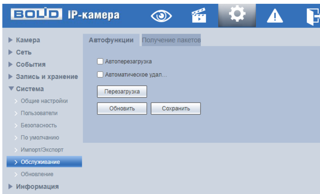
Рисунок 7.115 – Вкладка «Автофункции»
