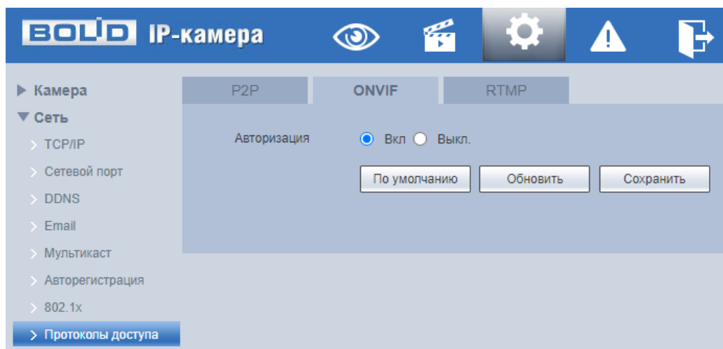
Рисунок 7.62 – Вкладка «ONVIF»
