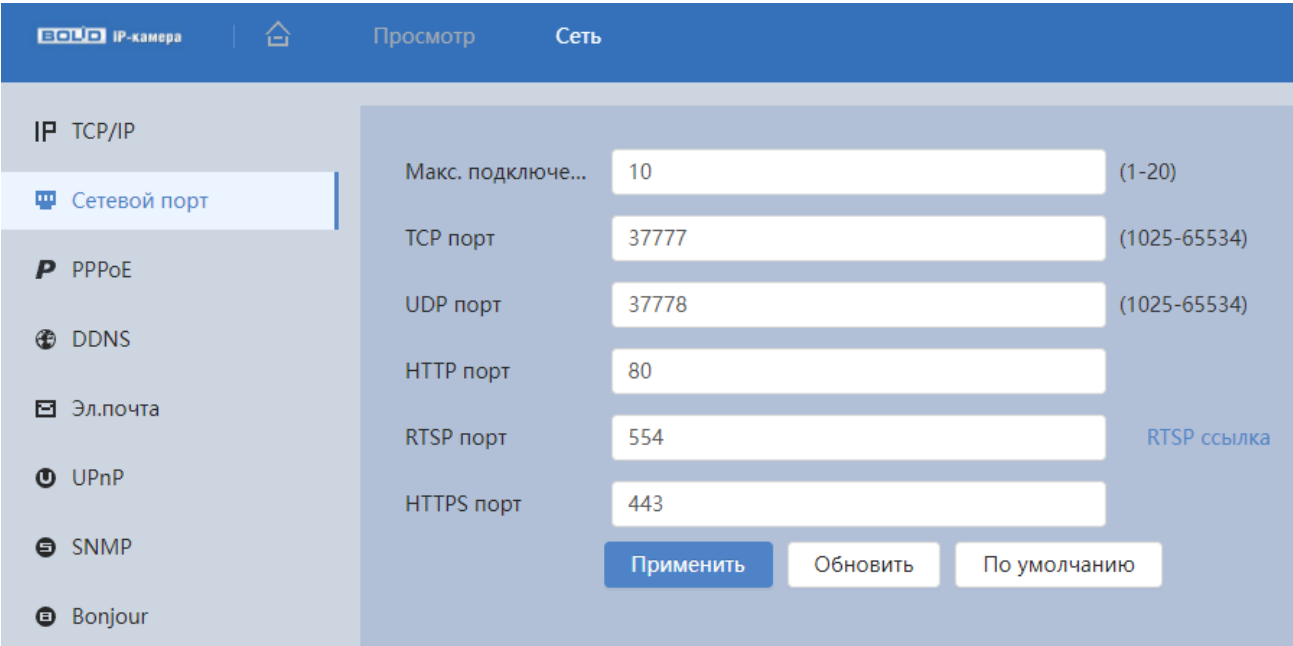
Рисунок 8.6 – Подпункт меню «Сетевой порт»
