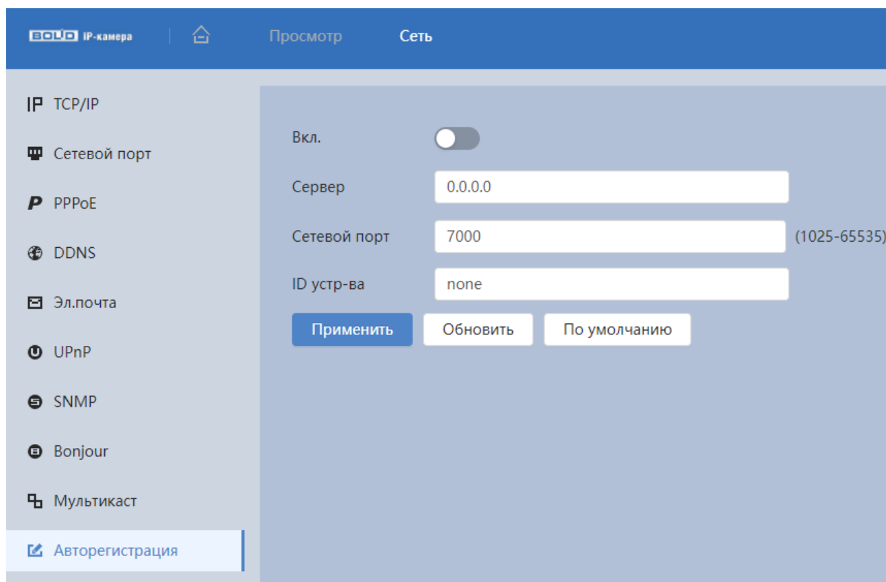
Рисунок 8.16 – Подпункт меню «Авторегистрация»
