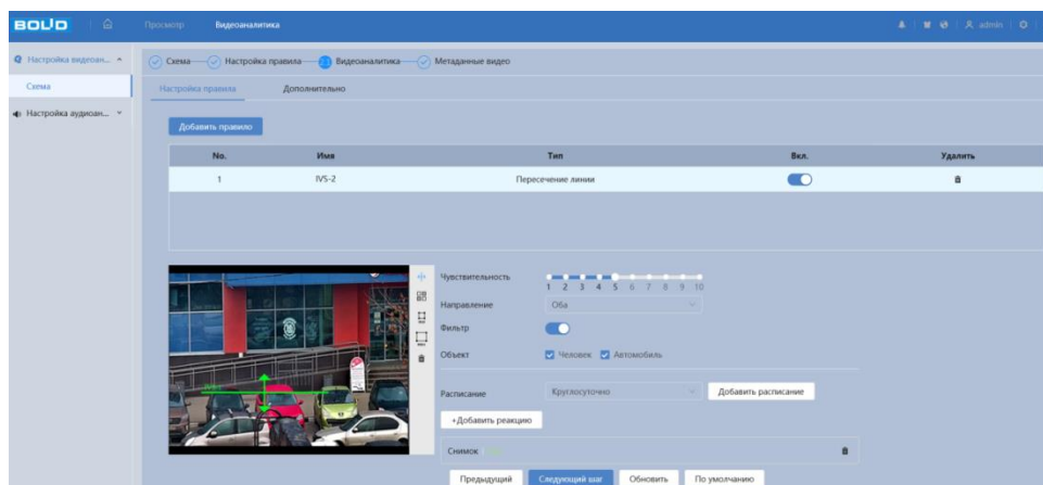
Рисунок 7.28 – Создание правила видеоаналитики «Пересечение линии»
