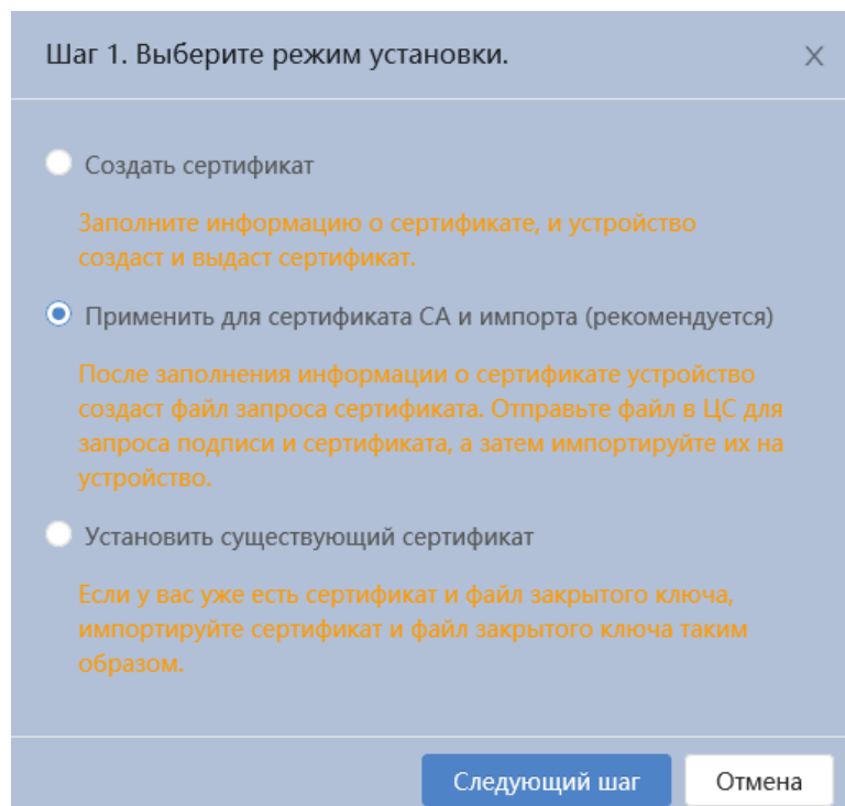
Рисунок 7.152 – Вкладка «Сертификат устройства»: Установка сертификата устройства, шаг 1
