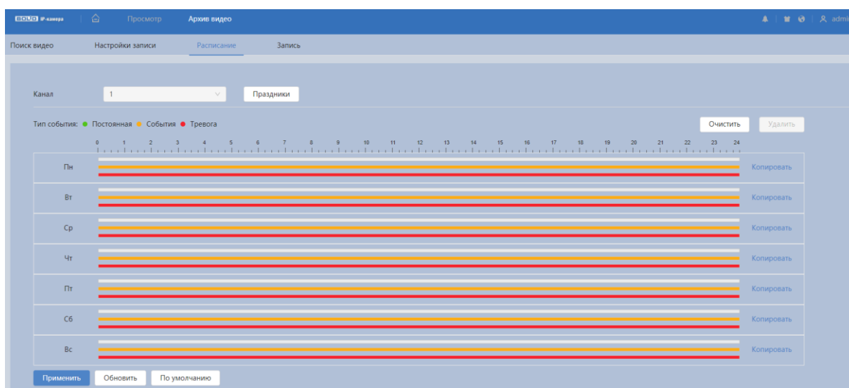
Рисунок 7.124 – Вкладка «Расписание»
