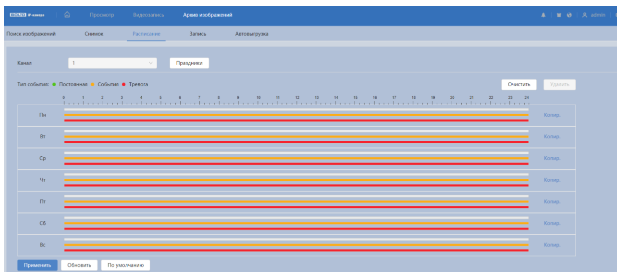
Рисунок 7.130 – Вкладка «Расписание»
