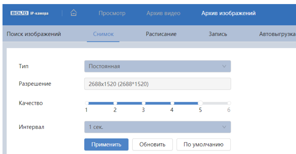
Рисунок 7.129 – Вкладка «Снимок»
