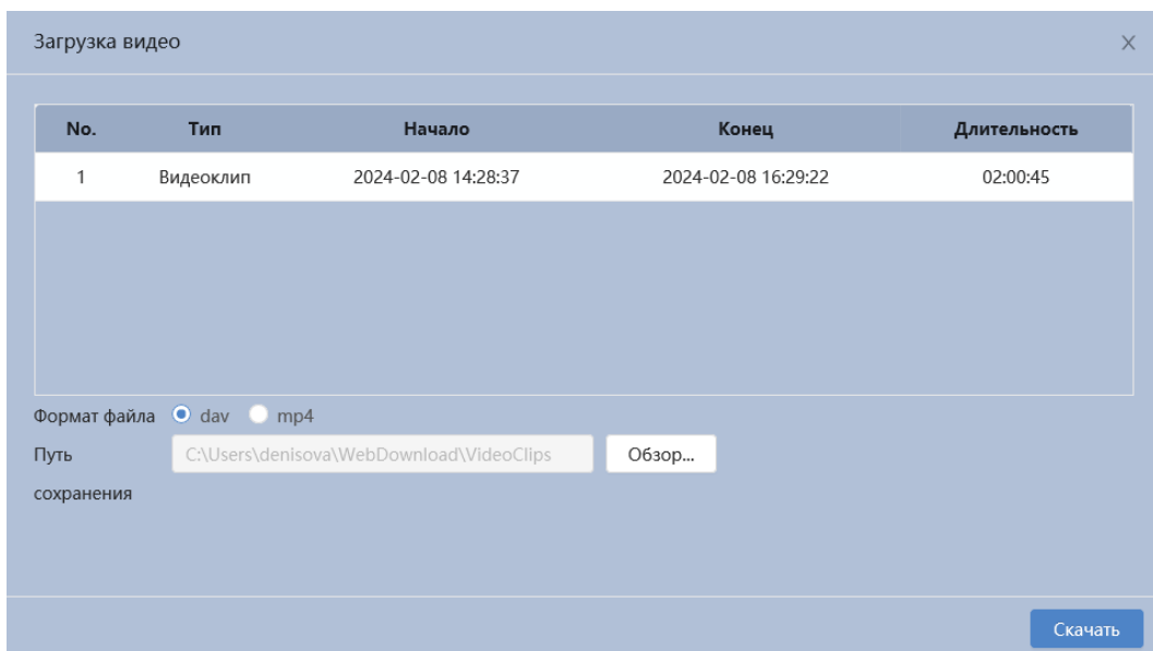
Рисунок 7.122 – Загрузка видео
