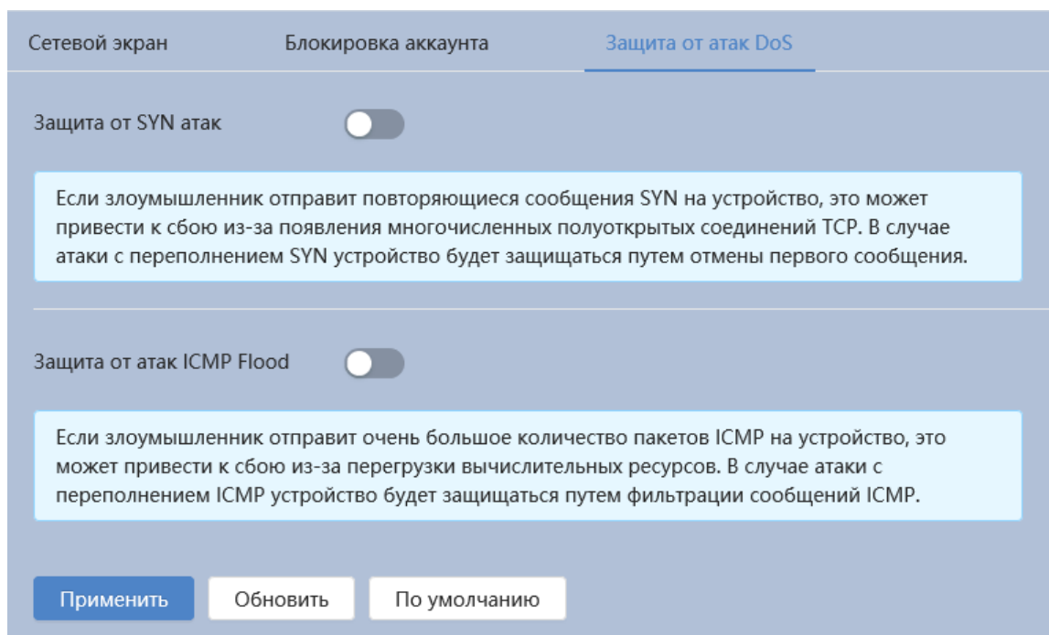
Рисунок 7.149 – Вкладка «Защита от атак DoS»
