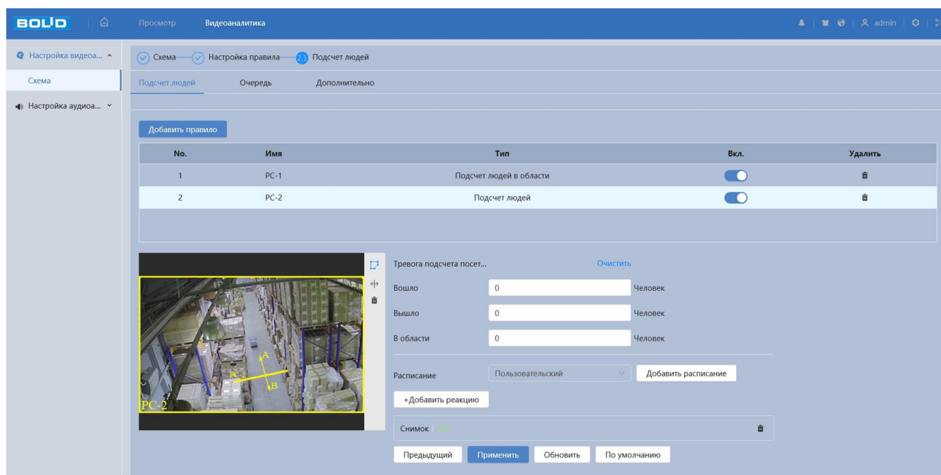
Рисунок 7.37 – Создание правила подсчета людей «Подсчет людей»
