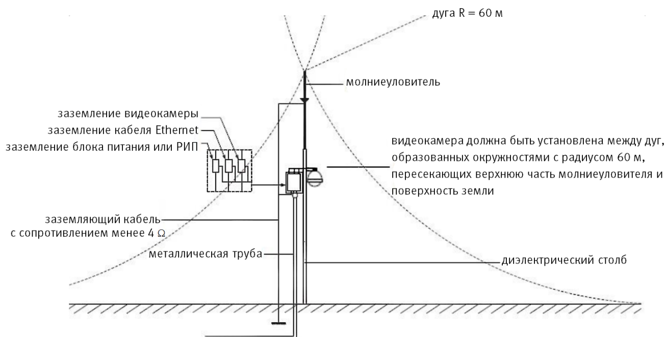
Рисунок 6.13 – Установка молниеотвода
