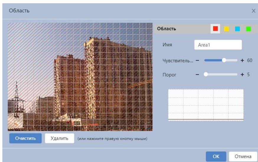
Рисунок 7.92 – Вкладка «Обнаружение движения: Область»
