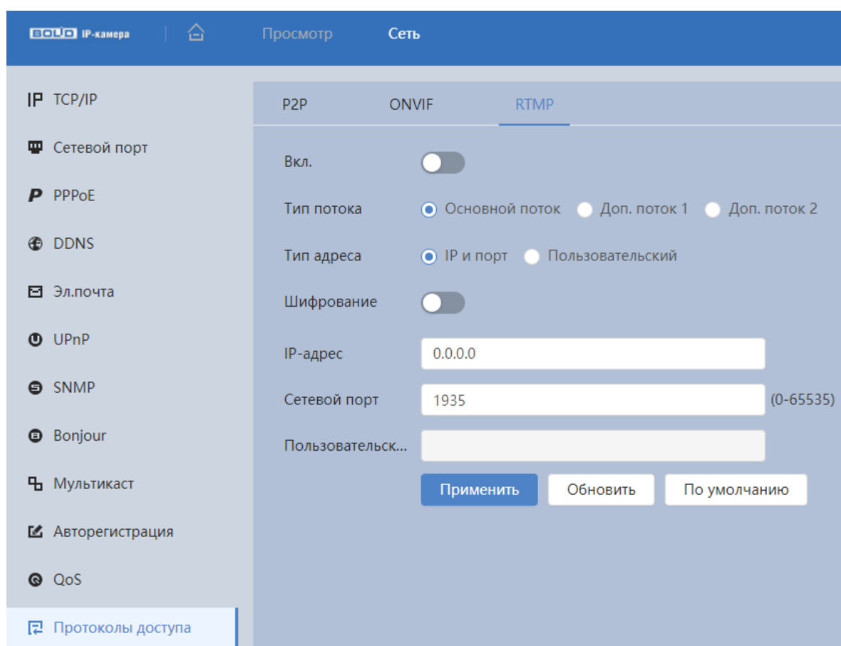
Рисунок 8.21 – Вкладка «RTMP»
