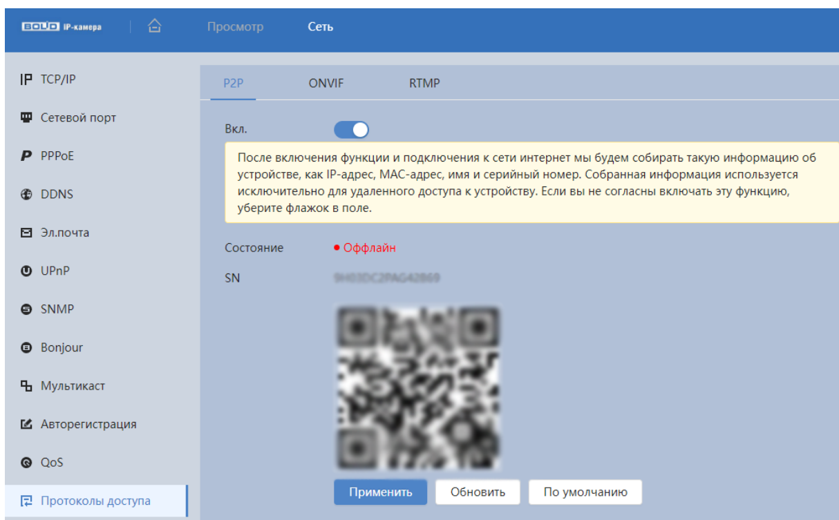
Рисунок 8.19 – Вкладка «P2P»
