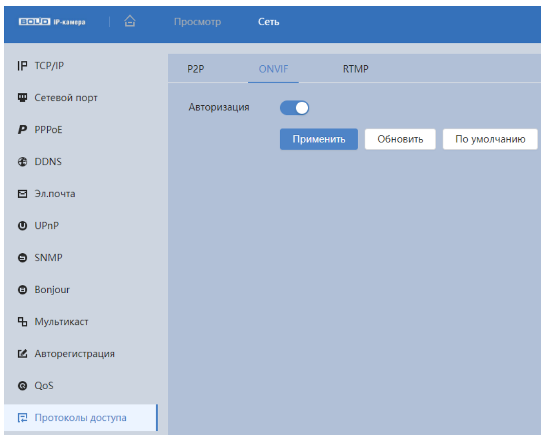
Рисунок 8.20 – Вкладка «ONVIF»
