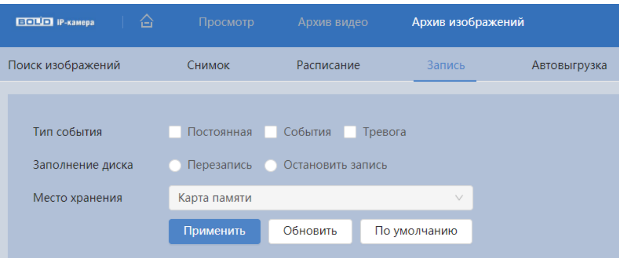
Рисунок 7.132 – Вкладка «Запись»
