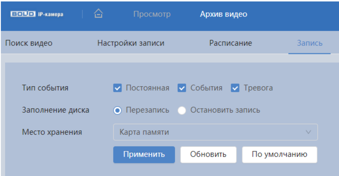
Рисунок 7.126 – Вкладка «Запись»
