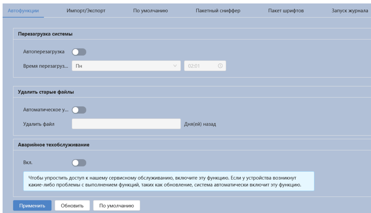
Рисунок 7.112 – Вкладка «Автофункции»
