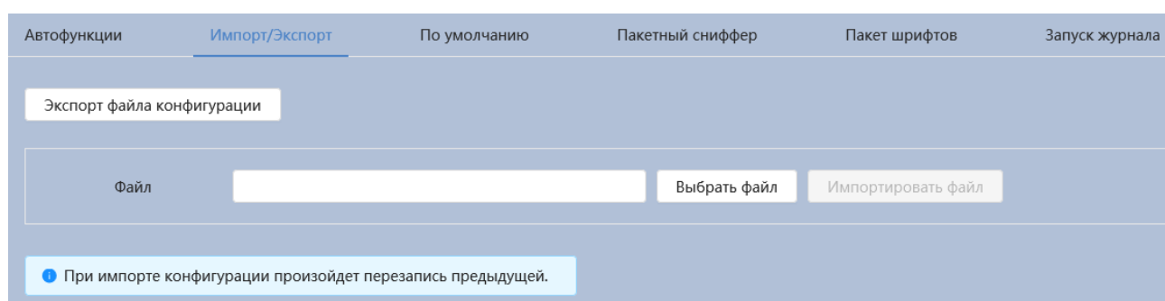
Рисунок 7.113 – Вкладка «Импорт/Экспорт»
