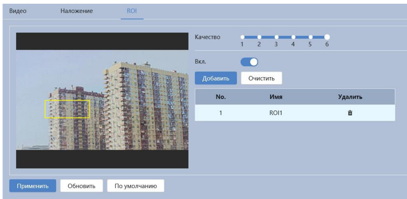
Рисунок 7.80 – Вкладка «ROI»
