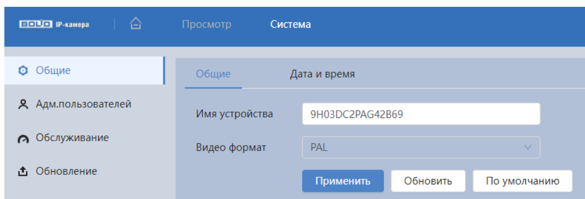
Рисунок 7.102 – Вкладка «Общие»
