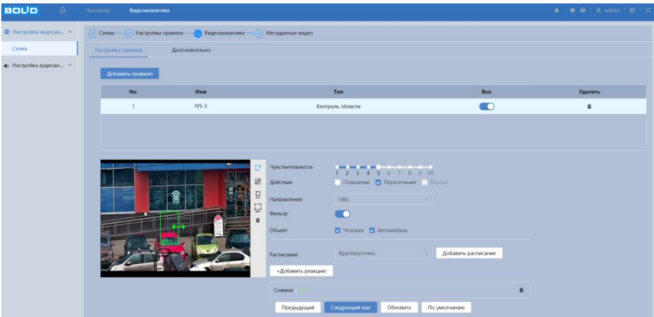
Рисунок 7.29 – Создание правила видеоаналитики «Контроль области»
