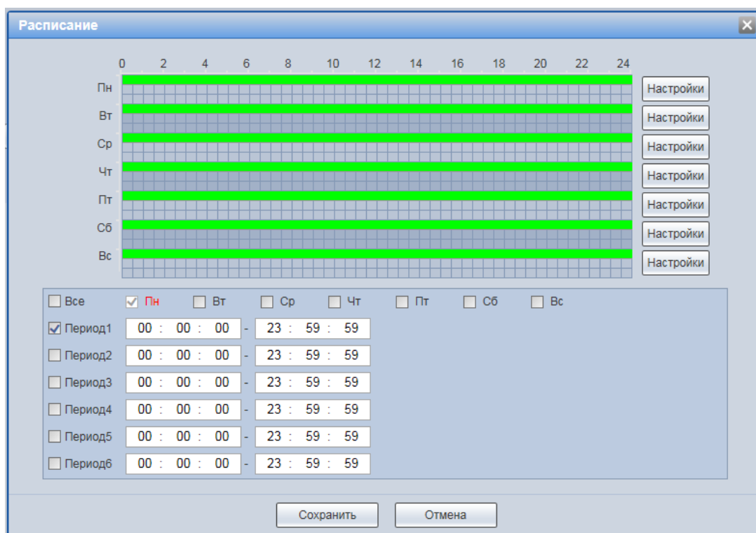
Рисунок 7.70 – Вкладка «Изменение сцены»: Расписание
