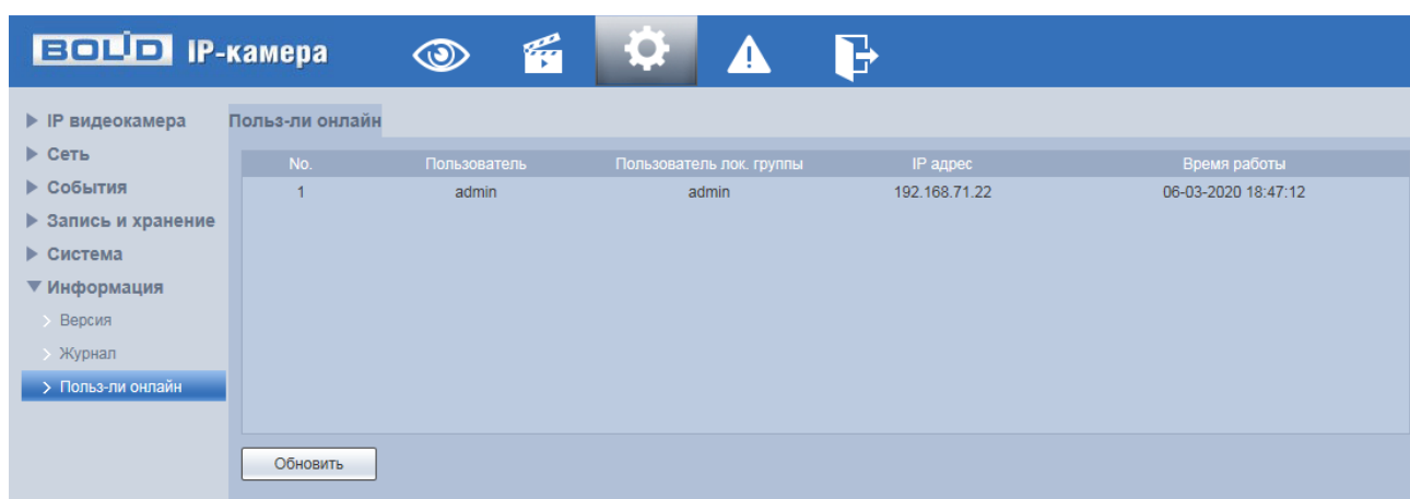
Рисунок 7.121 – Пункт меню «Пользователи онлайн»
