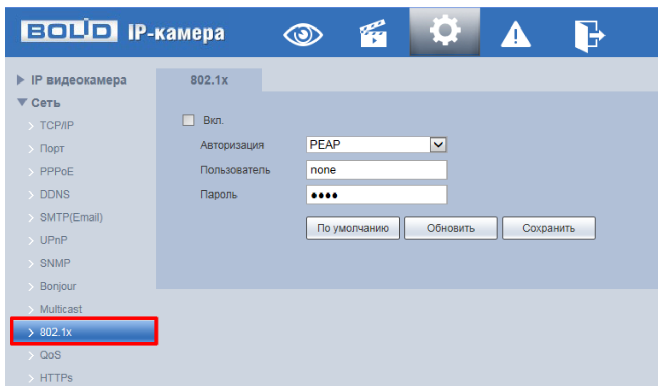
Рисунок 7.58 – Подпункт меню «802.1x»
