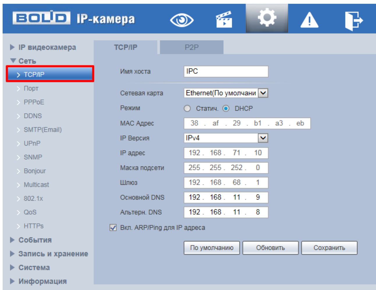
Рисунок 7.44 – Подпункт меню «TCP/IP»
