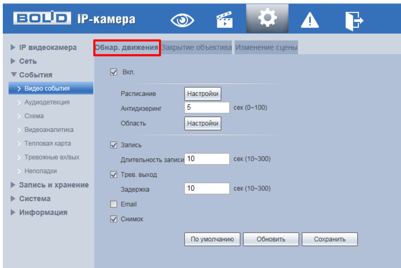
Рисунок 7.65 - Вкладка «Обнаружение движения»
