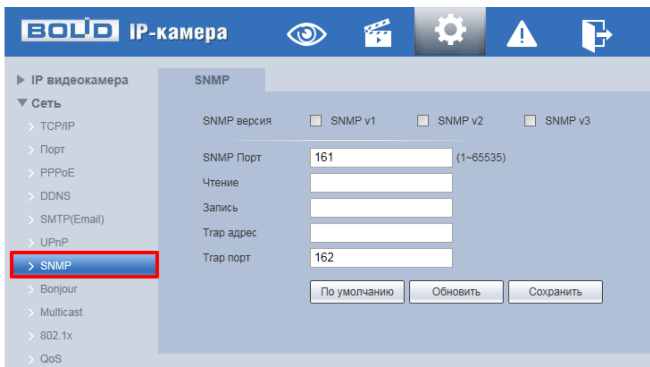
Рисунок 7.55 – Подпункт меню «SNMP»
