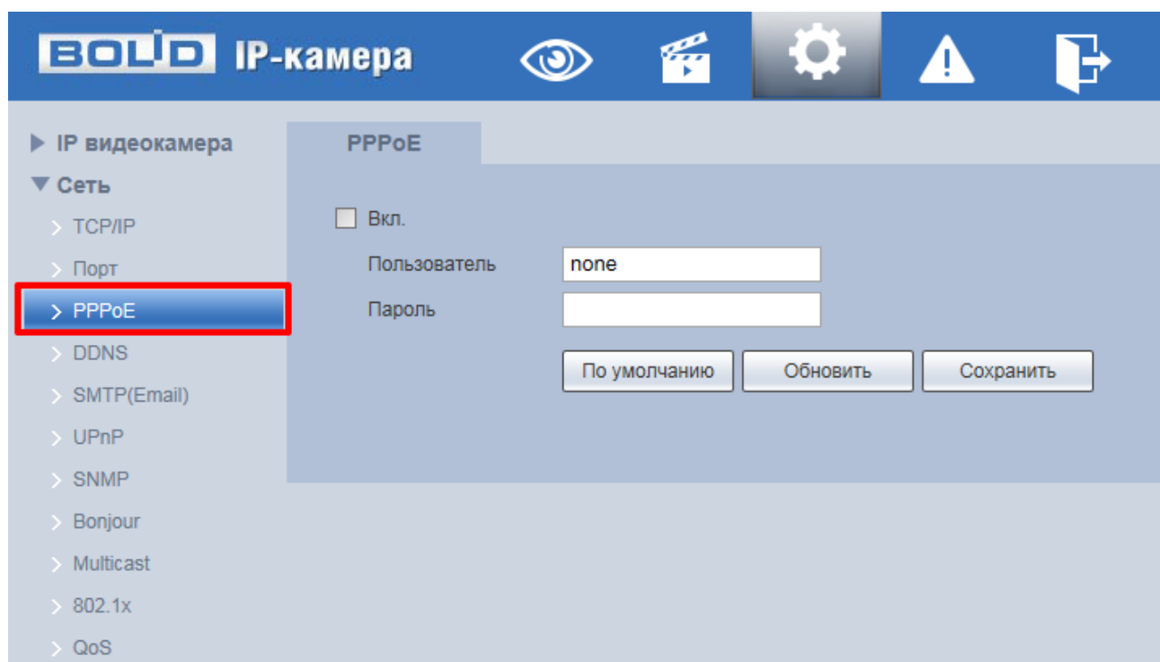
Рисунок 7.48 – Подпункт меню «PPPoE»
