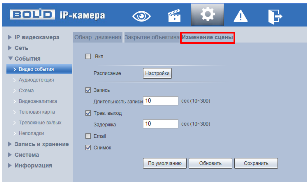
Рисунок 7.69 – Вкладка «Изменение сцены»
