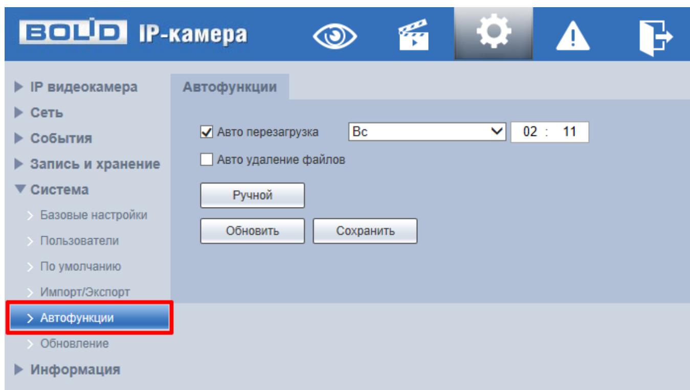
Рисунок 7.113 – Подпункт меню «Автофункции»
