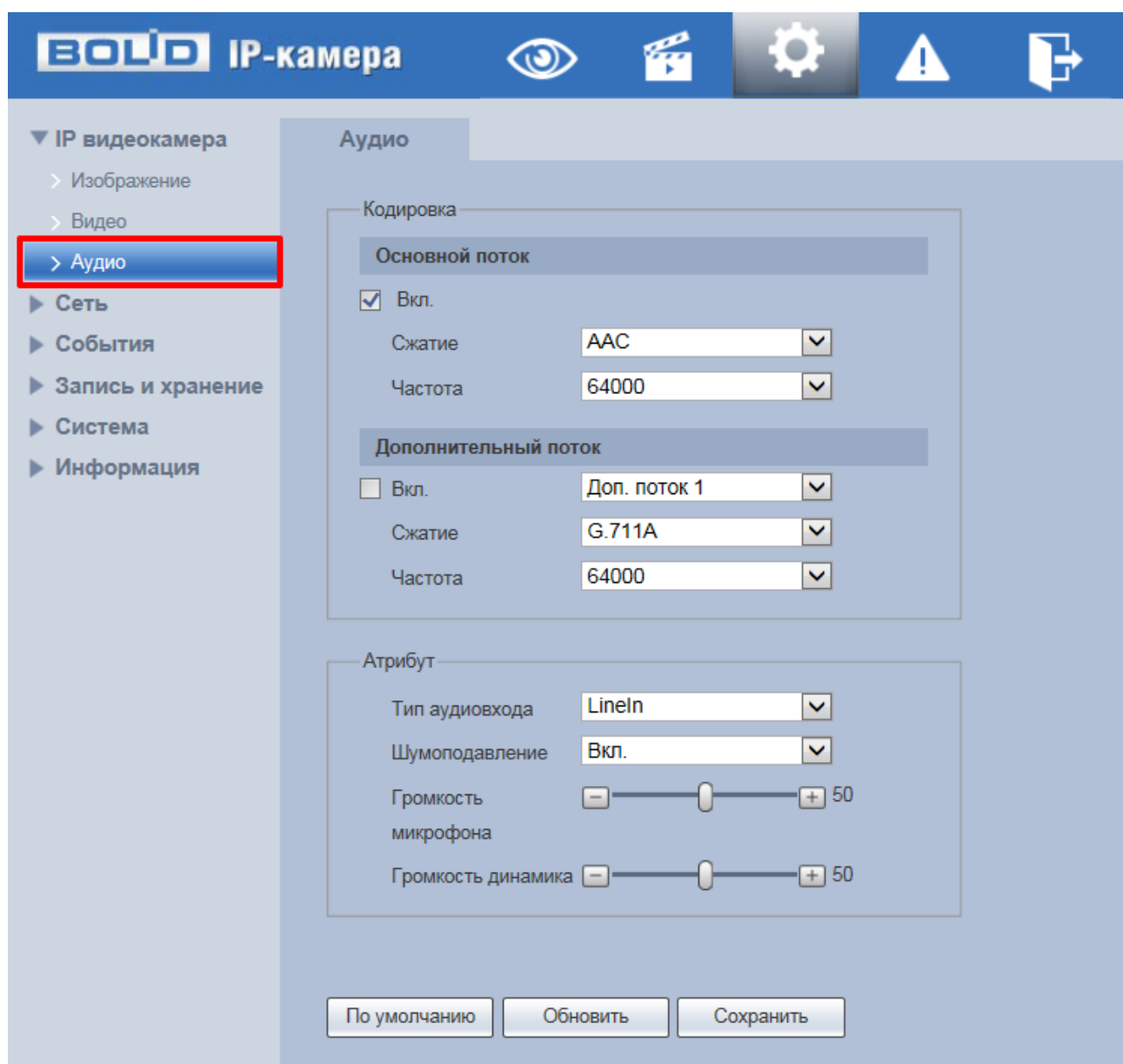
Рисунок 7.41 - Подпункт меню «Аудио»
