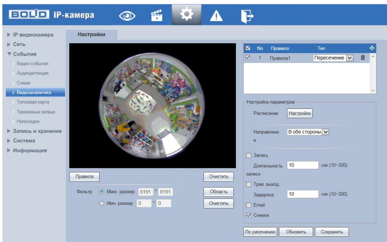
Рисунок 7.74 - Подпункт меню «Видеоаналитика»: Пересечение линии
