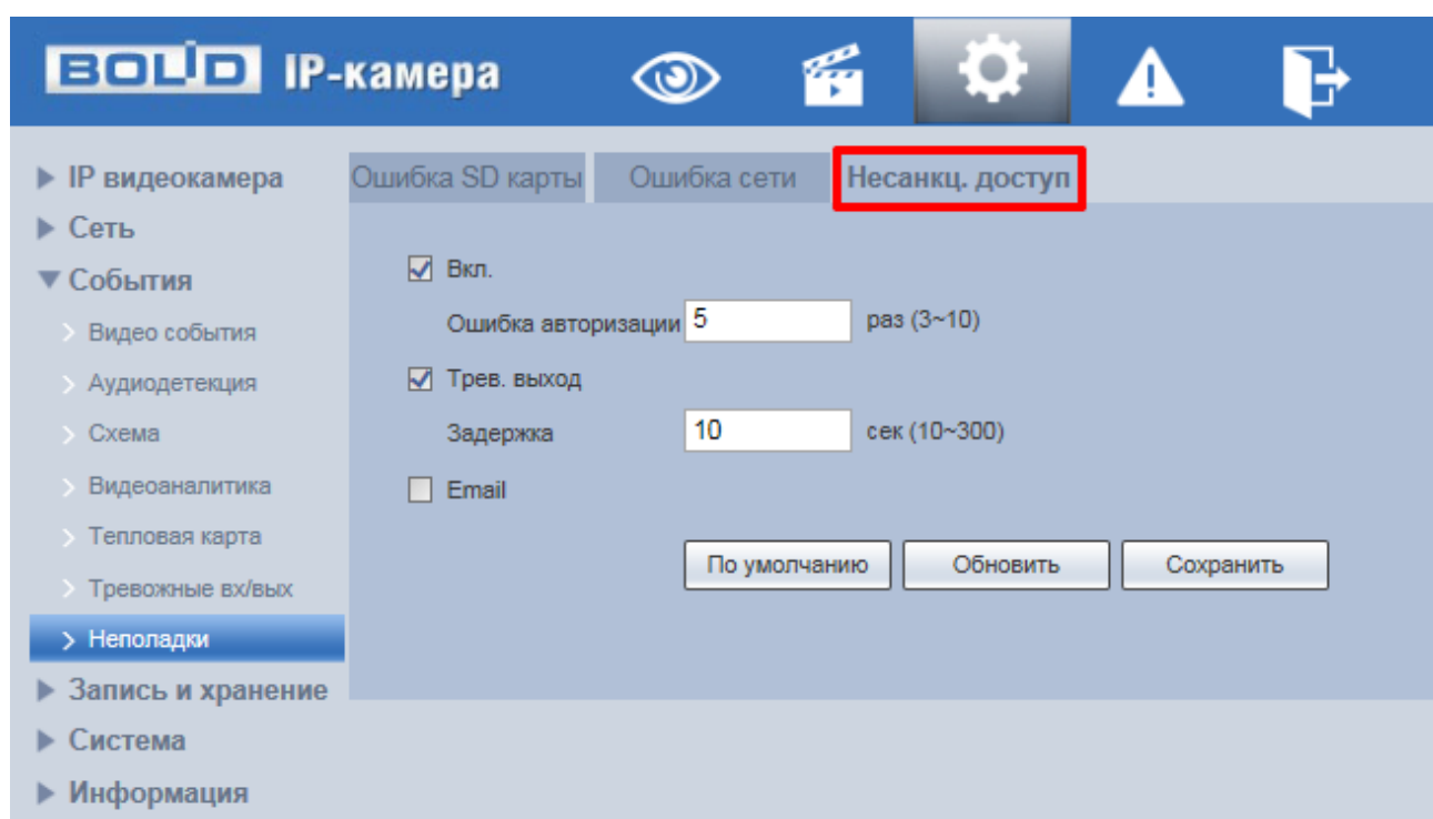
Рисунок 7.85 – Вкладка «Несанкционированный доступ»
