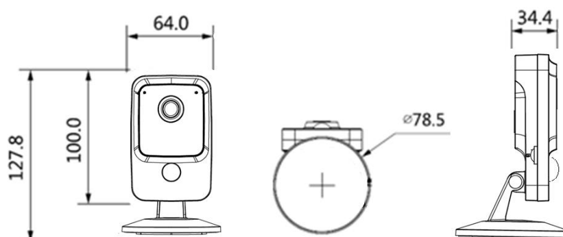
Рисунок 4.2 – Габаритные размеры видеокамеры
