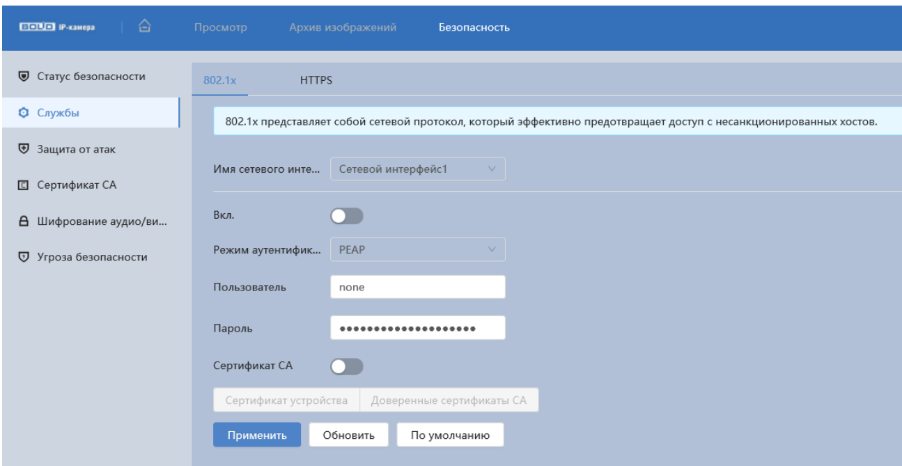
Рисунок 7.132 – Вкладка «Службы: 802.1x»
