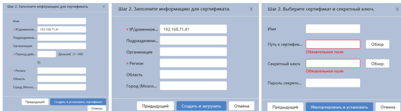
Рисунок 7.141 – Вкладка «Сертификат устройства»: Шаг 2. Информация для сертификата
