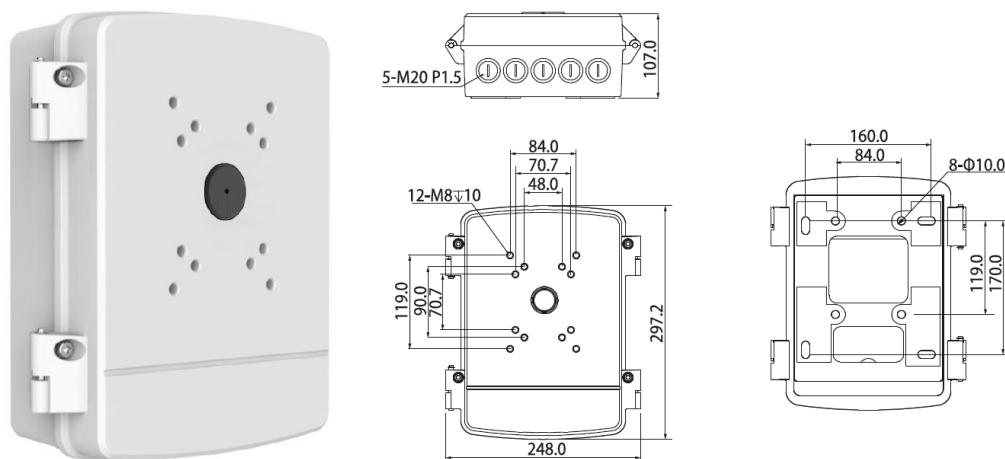
Рисунок 5.4 – Монтажная коробка BR-203
