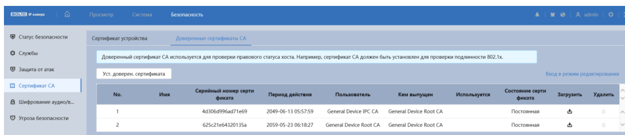
Рисунок 7.142 – Вкладка «Доверенные сертификаты CA»
