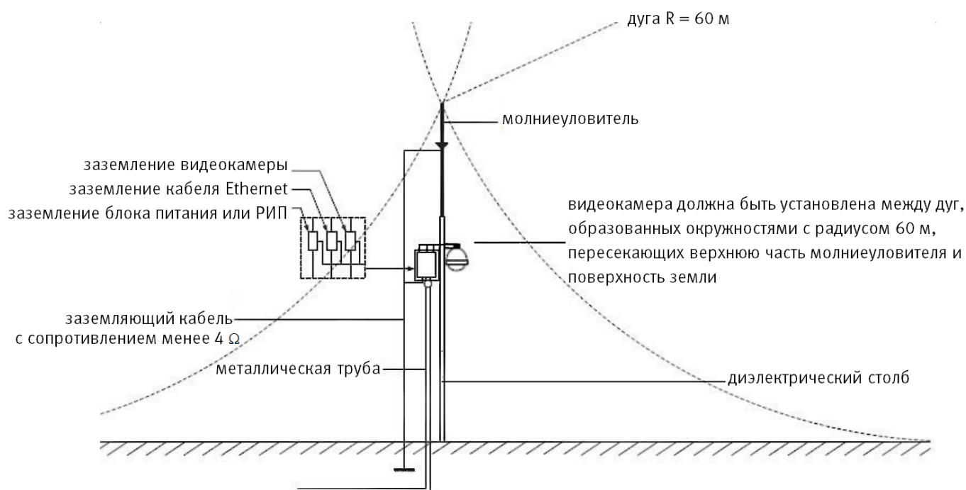
Рисунок 6.13 – Установка молниеотвода
