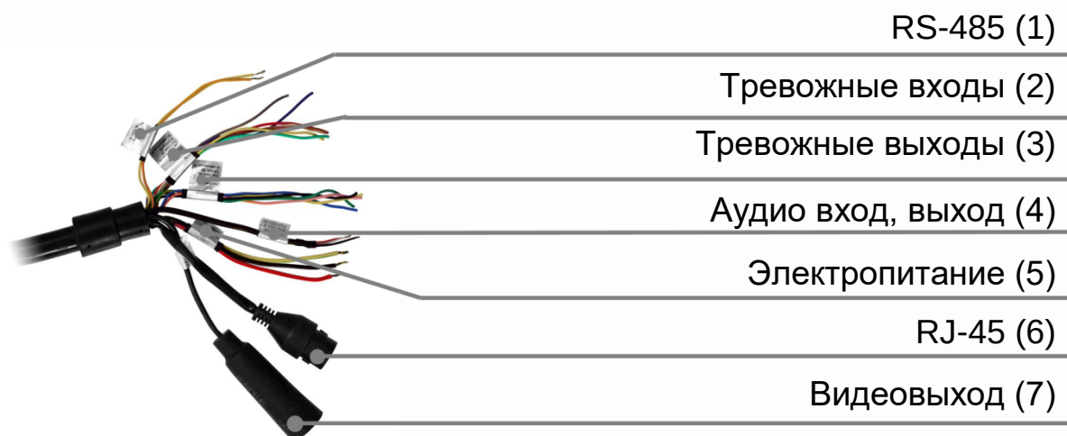
Рисунок 6.1 – Группы концевой раскладки кабеля видеокамеры
