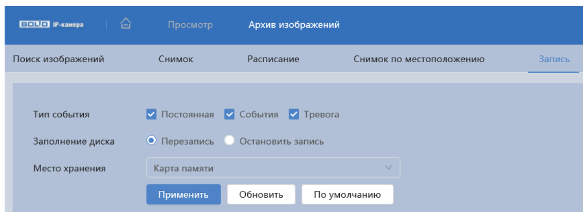
Рисунок 7.138 – Вкладка «Запись»
