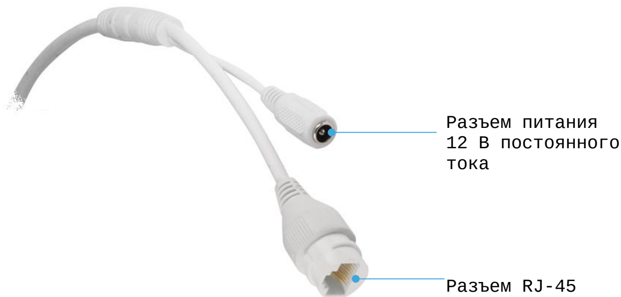
Рисунок 6.1 – Кабель видеокамеры
