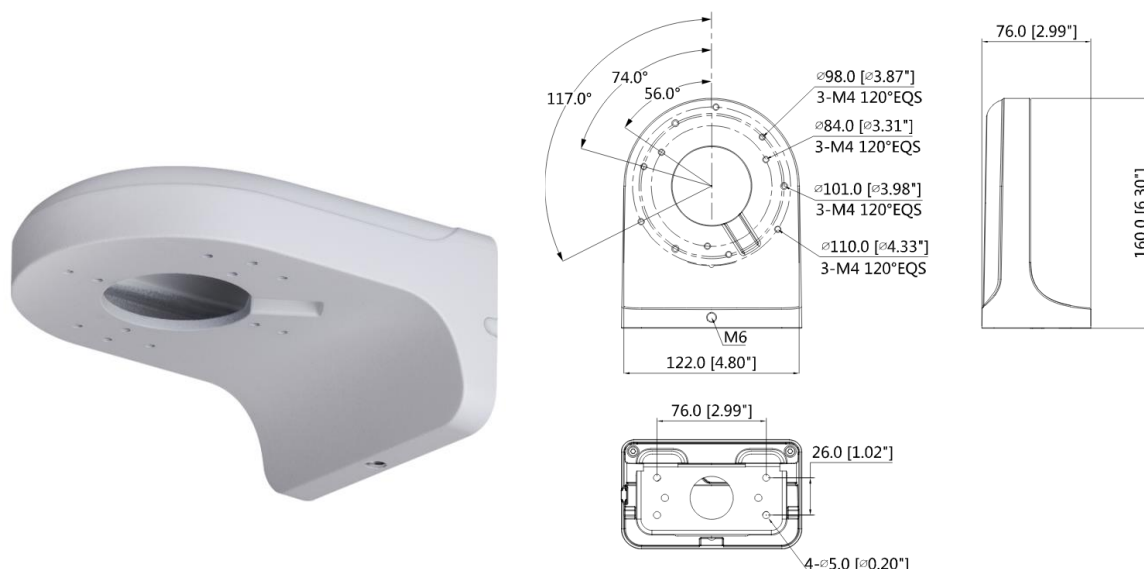
Рисунок 5.6 – Кронштейн BR-106
