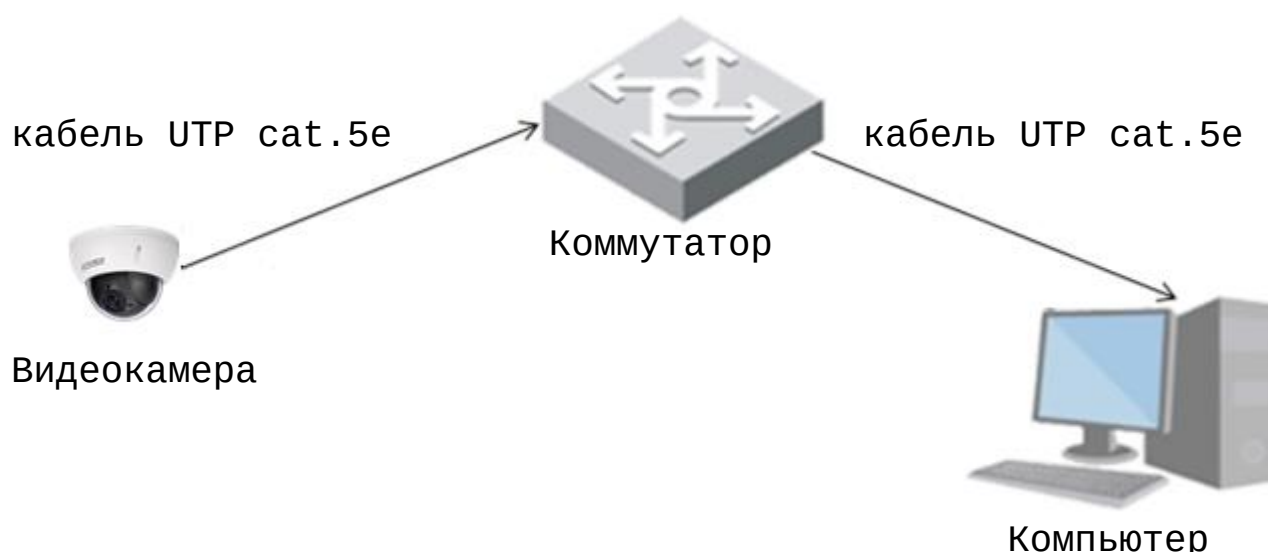
Рисунок 6.3 – Схема подключения видеокамеры к компьютеру через коммутатор
