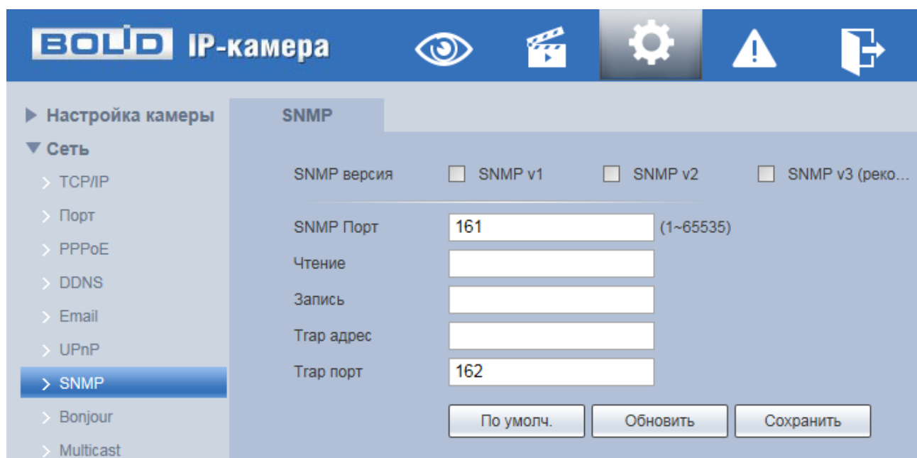
Рисунок 7.61 — Подпункт меню «SNMP»
