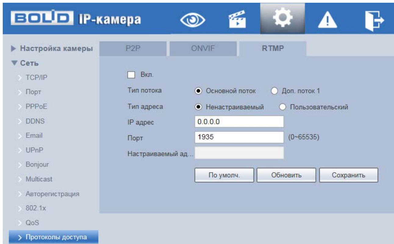
Рисунок 7.69 — Вкладка «RTMP»
