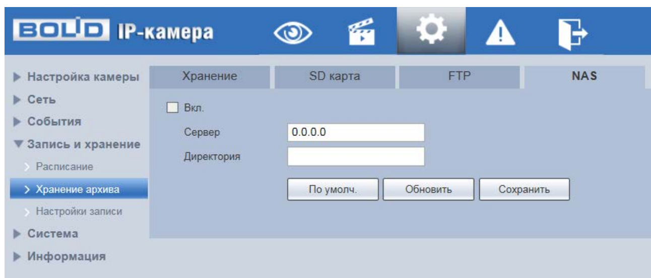
Рисунок 7.104 — Вкладка «NAS»
