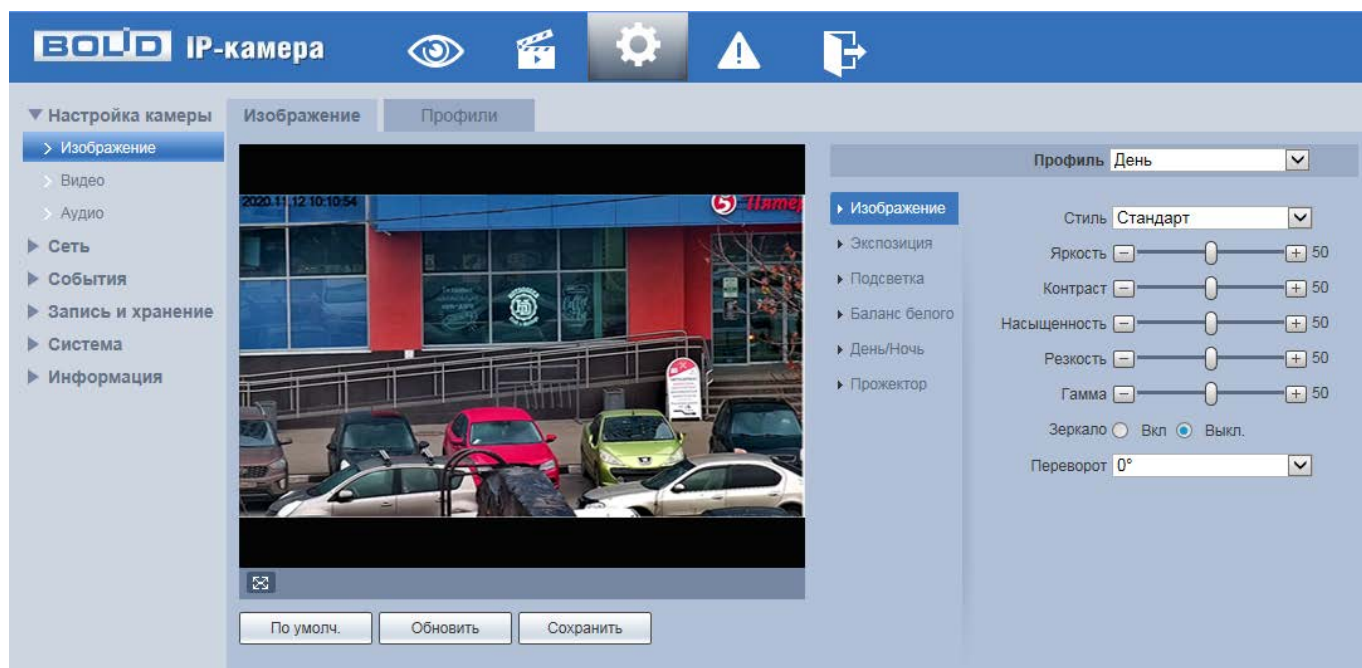
Рисунок 7.27 — Вкладка «Изображение»
