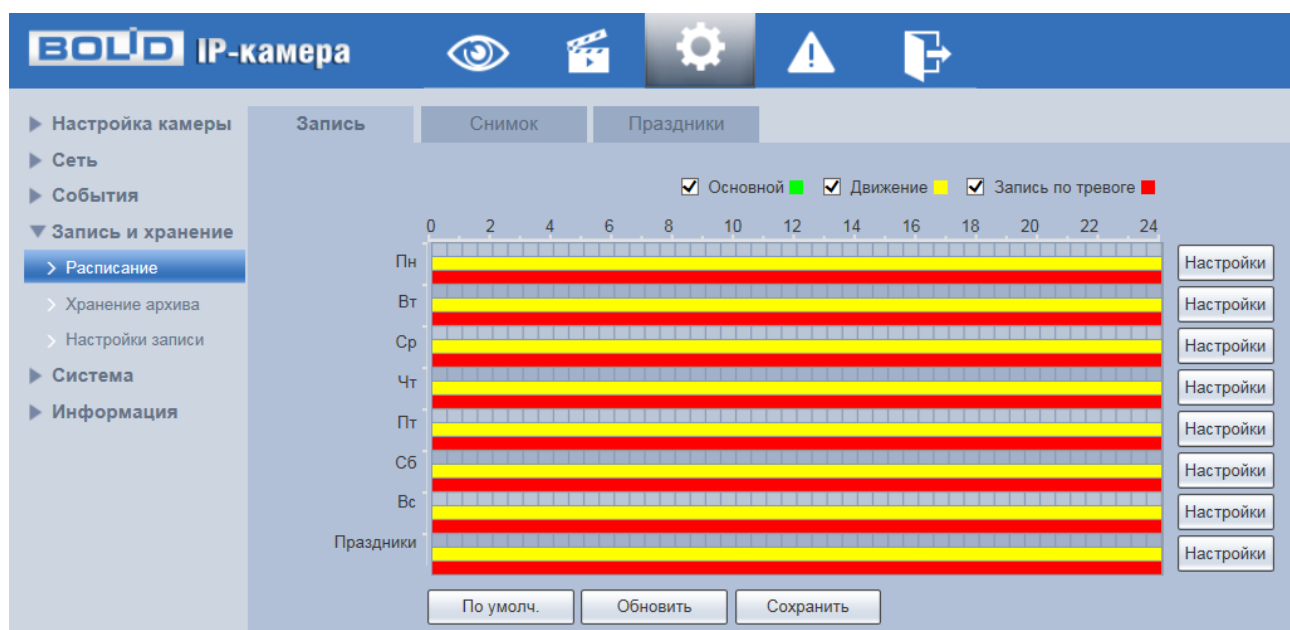
Рисунок 7.95 — Вкладка «Запись»
