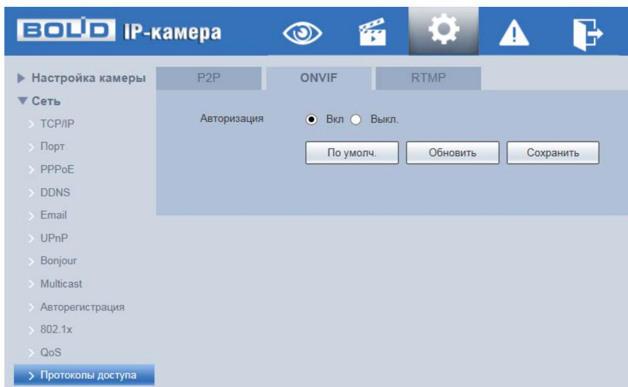
Рисунок 7.68 — Вкладка «ONVIF»
