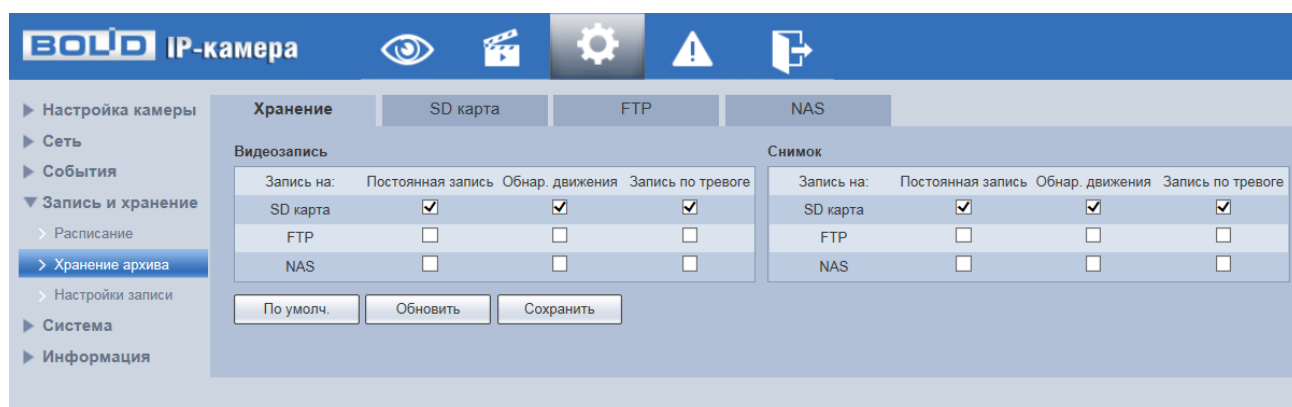
Рисунок 7.101 — Вкладка «Хранение»
