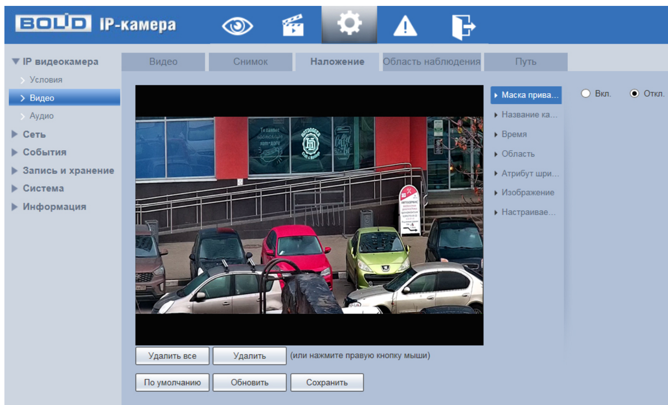
Рисунок 7.40 — Вкладка «Наложение»
