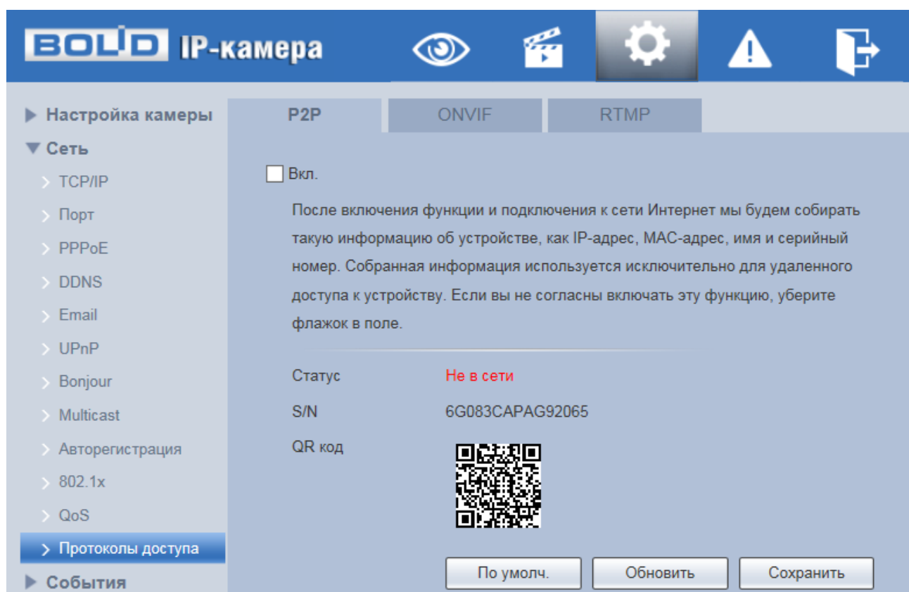
Рисунок 7.67 — Вкладка «P2P»
