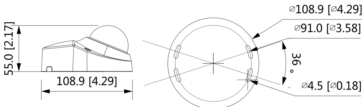
Рисунок 5.1 — Габаритные размеры видеокамеры
