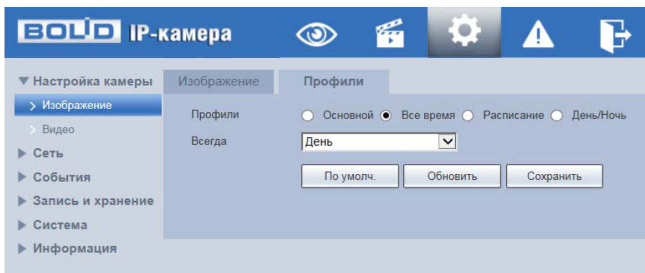
Рисунок 7.36 — Вкладка «Профили»
