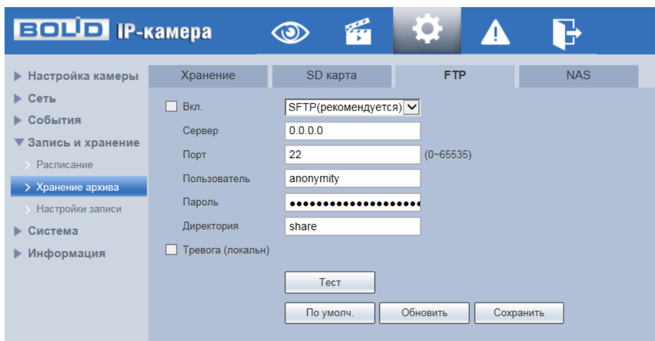
Рисунок 7.103 — Вкладка «FTP»
