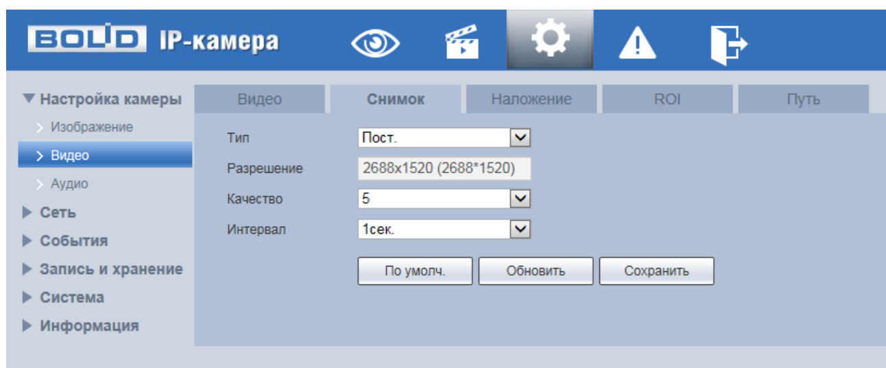
Рисунок 7.39 — Вкладка «Снимок»
