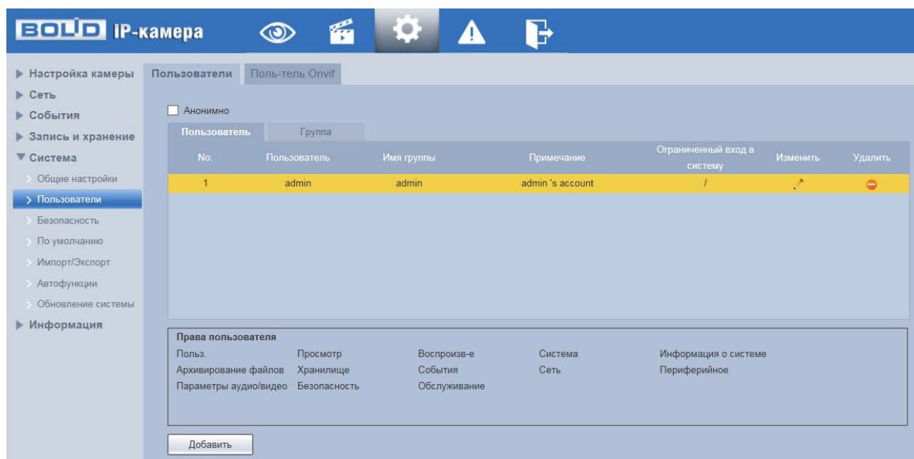
Рисунок 7.112 — Вкладка «Пользователи»
