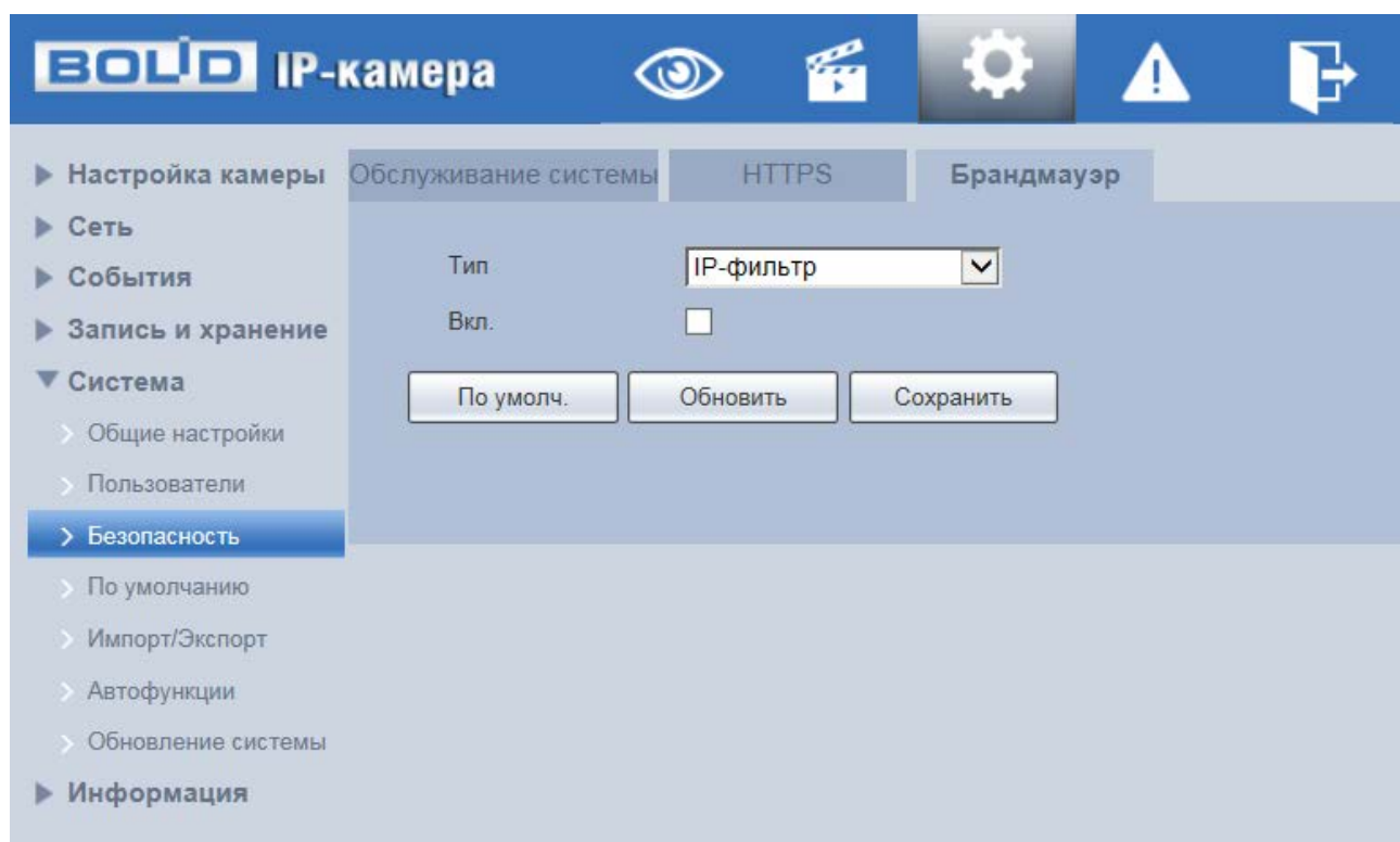
Рисунок 7.118 — Вкладка «Брандмауэр»
