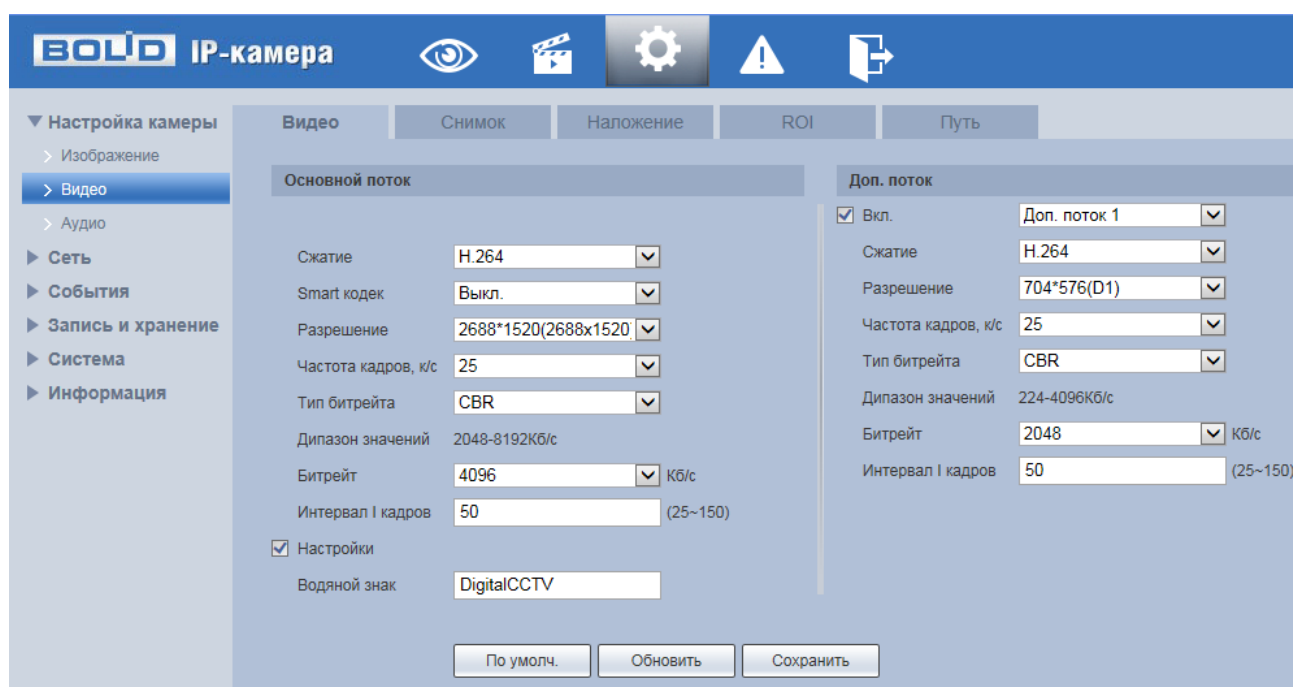
Рисунок 7.38 — Вкладка «Видео»
