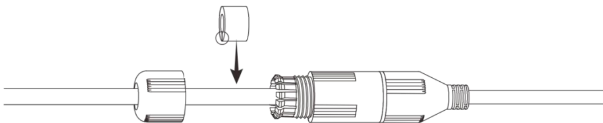
Рисунок 6.9 – Втулка герметичной кабельной муфты
