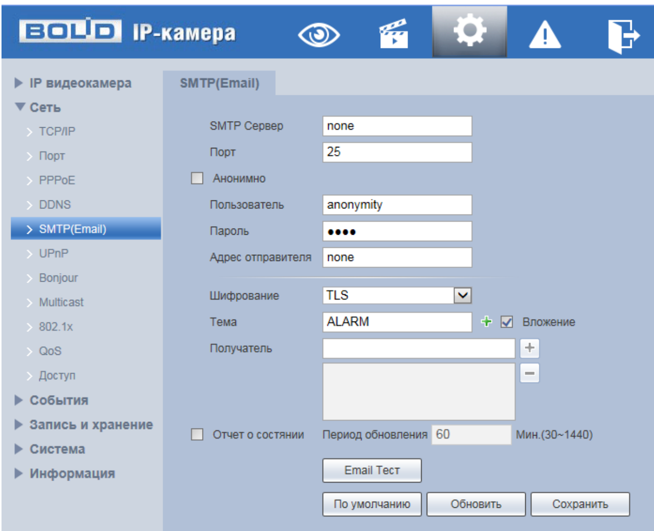
Рисунок 7.55 – Подпункт меню «SMTP»
