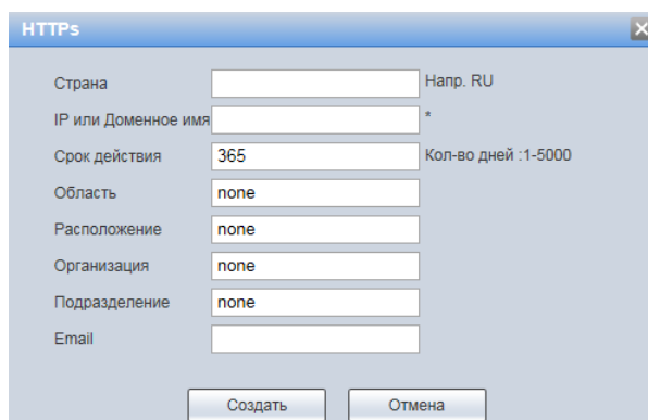
Рисунок 7.113 – Подпункт меню «HTTPS: Создать сертификат»
