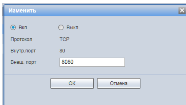
Рисунок 7.58 – Подпункт меню «UPnP»: Изменение перенаправления портов
