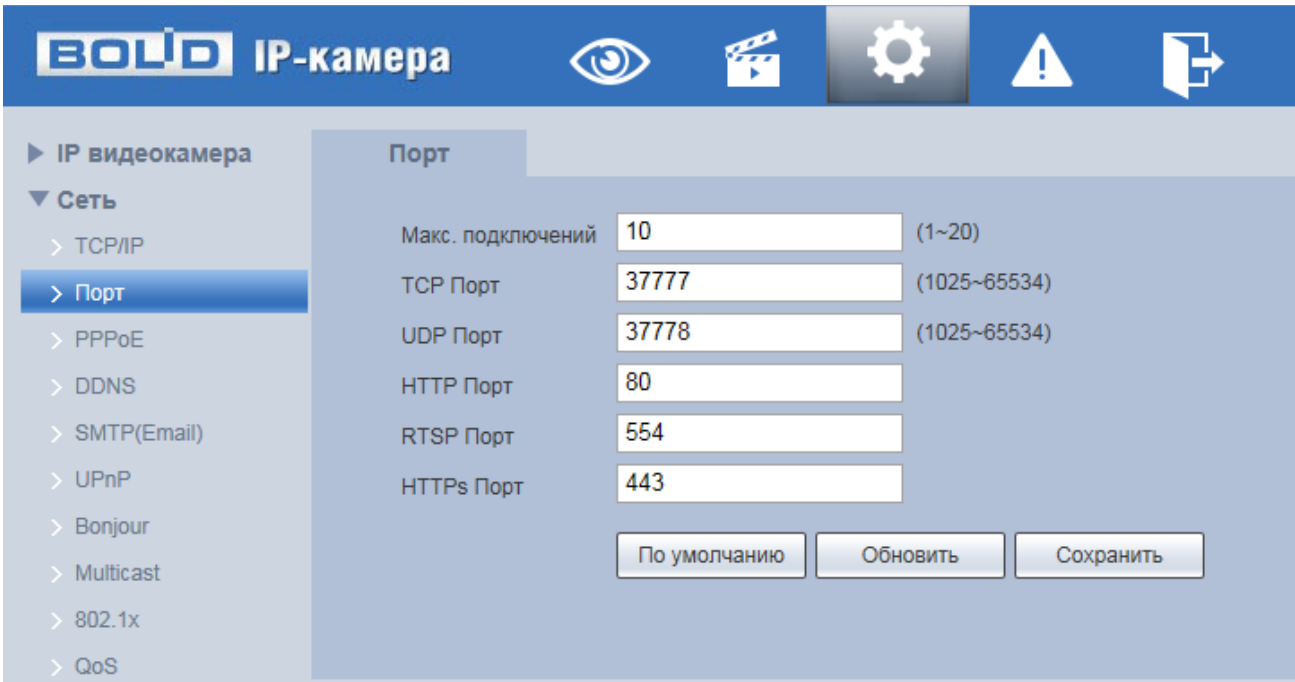
Рисунок 7.51 – Подпункт меню «Порт»
