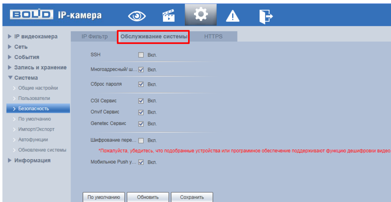
Рисунок 7.111 - Вкладка «Обслуживание системы»
