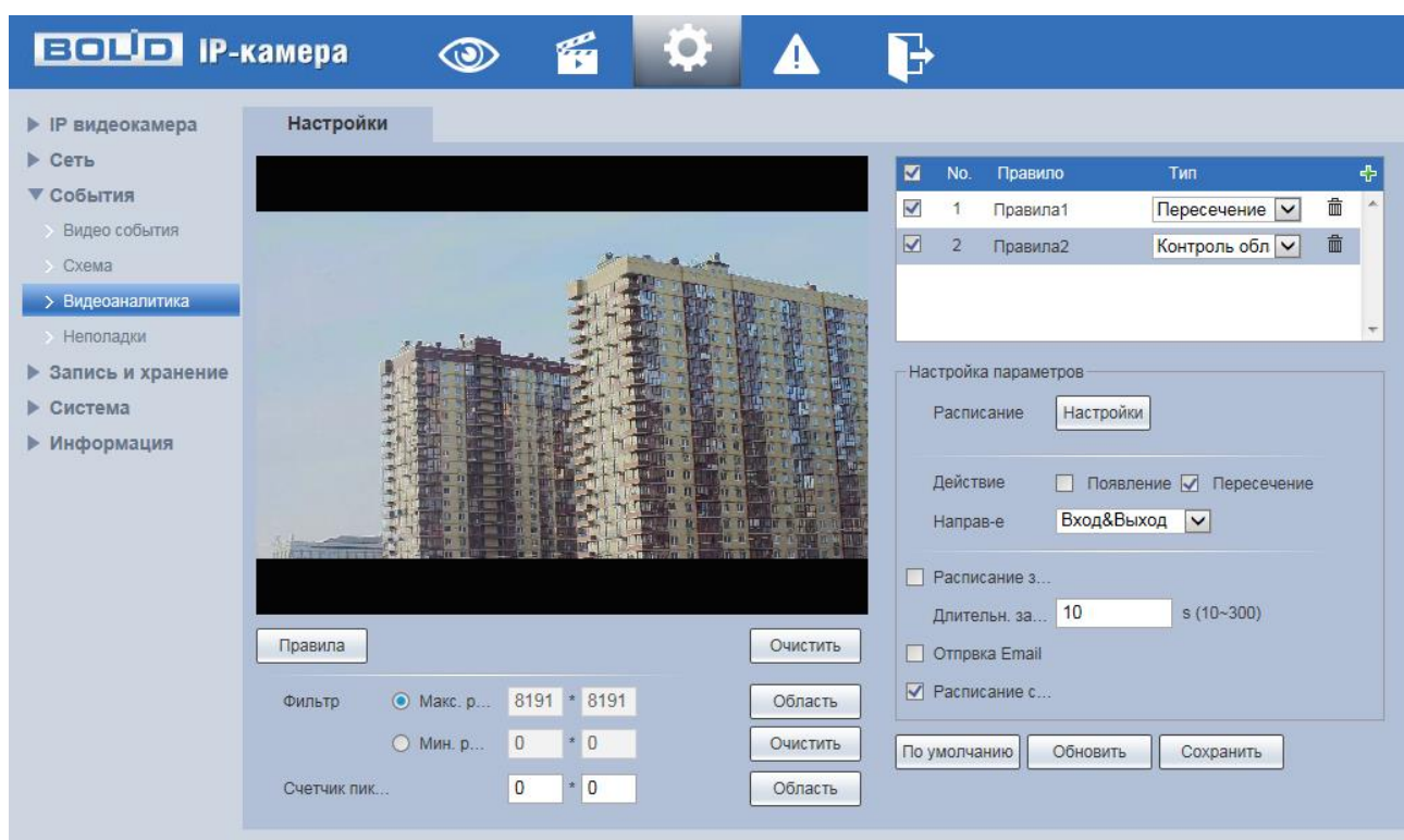
Рисунок 7.78 – Подпункт меню «Видеоаналитика»
