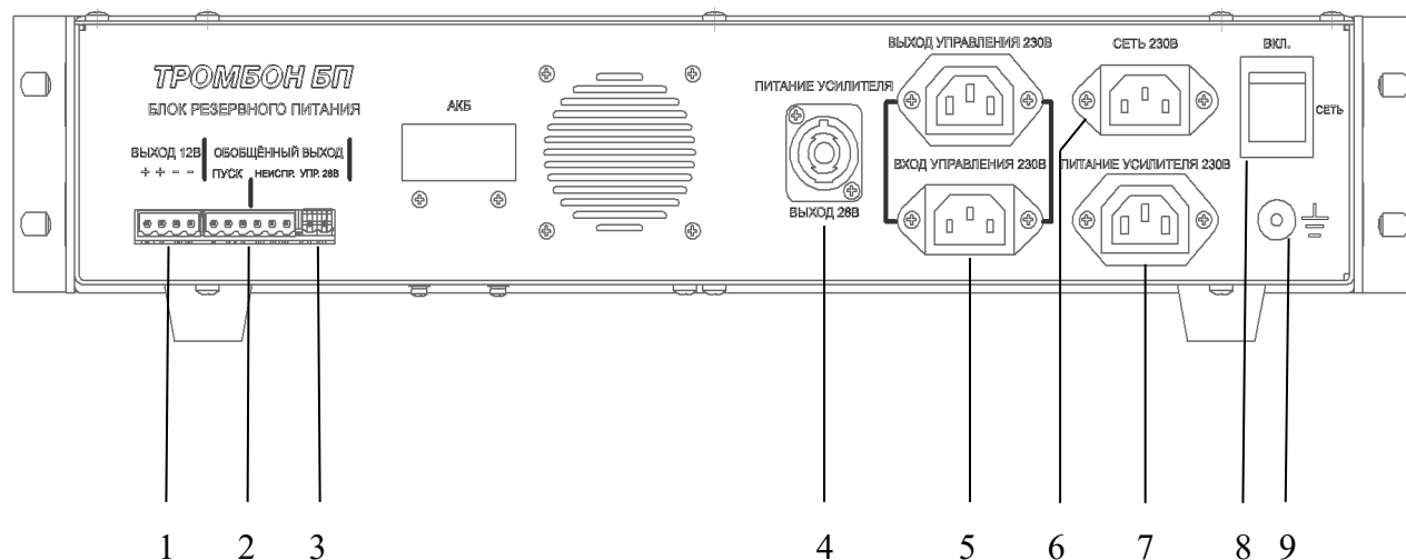
Рисунок 2 – Вид на заднюю панель прибора и расположение органов управления и коммутации
