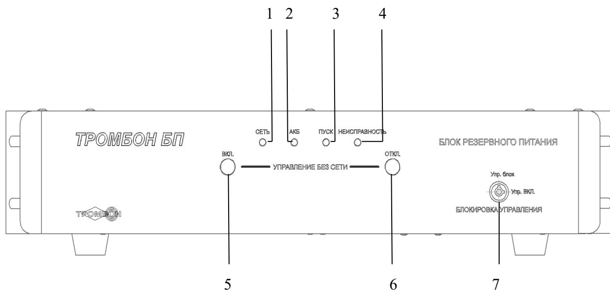
Рисунок 1 – Внешний вид прибора и расположение органов управления и индикации
