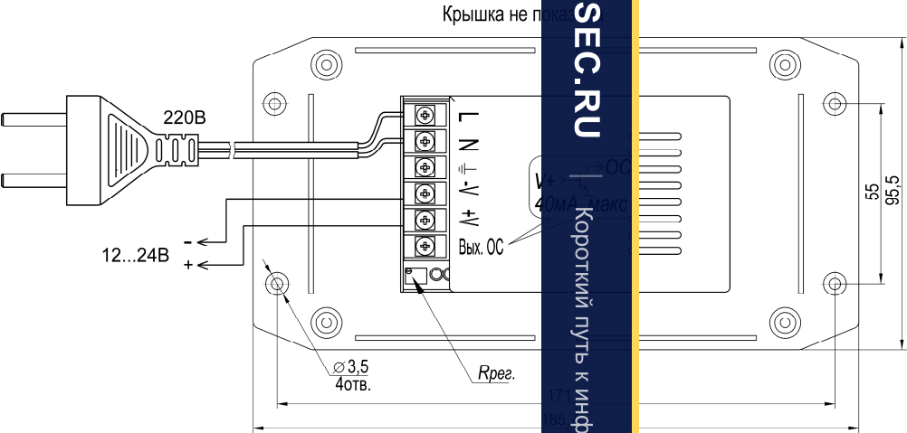
Рис.1 Устройство, габаритные и установочные размеры изделия
