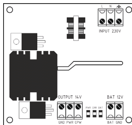
Рисунок 1. Внешний вид источника питания и назначение разъёмов
