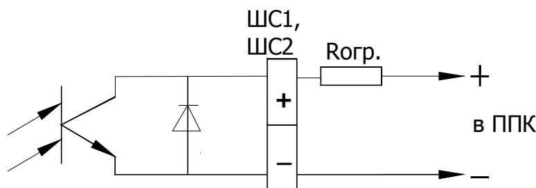
Рисунок 1 Схема подключения шлейфов сигнализации. Rогр. устанавливается в соответствии с документацией на ППК
