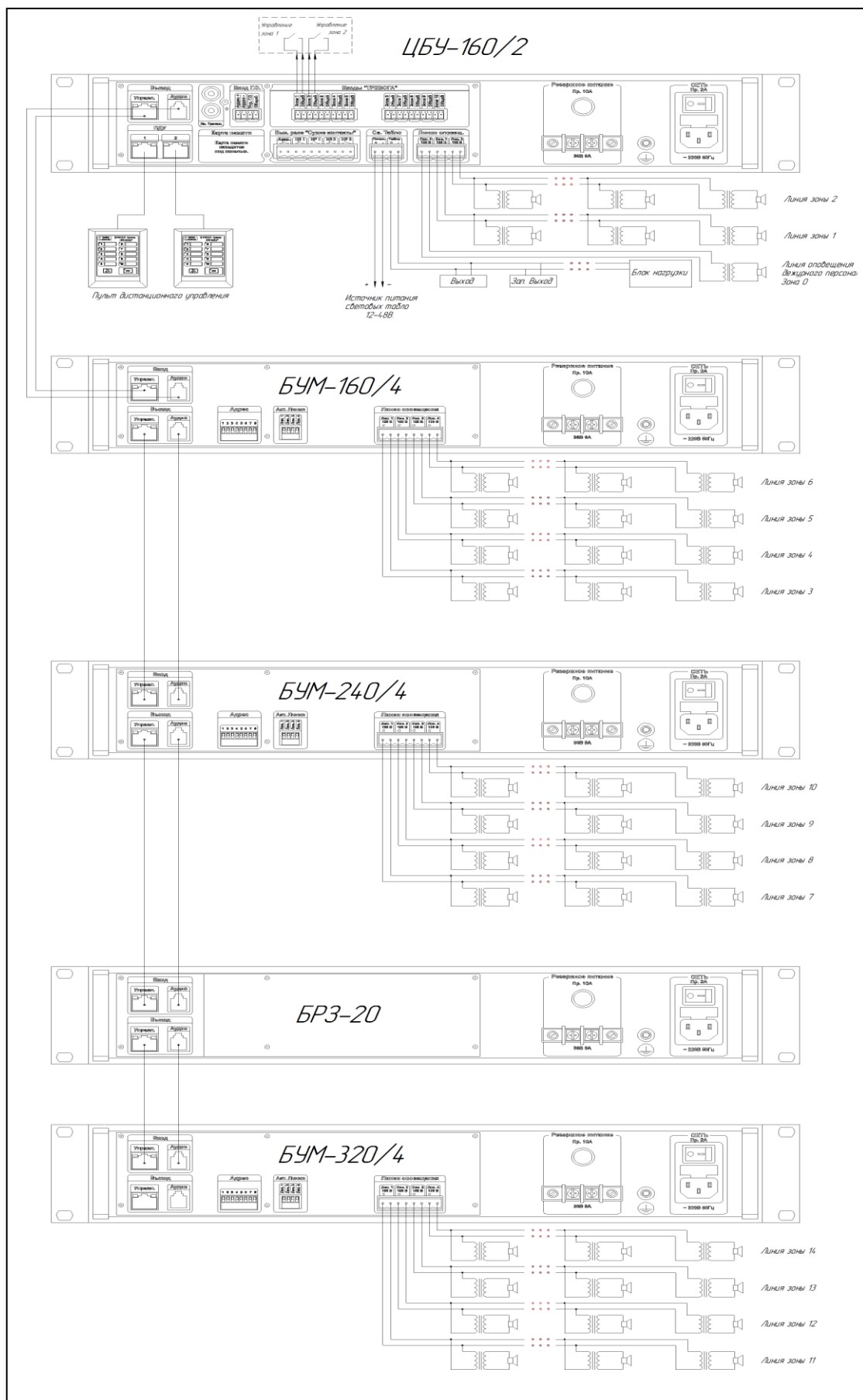
Рис.5. Типовая схема включения блока расширения зон БР3-20 системы автоматического речевого оповещения «РЕЧОР Гранд».
