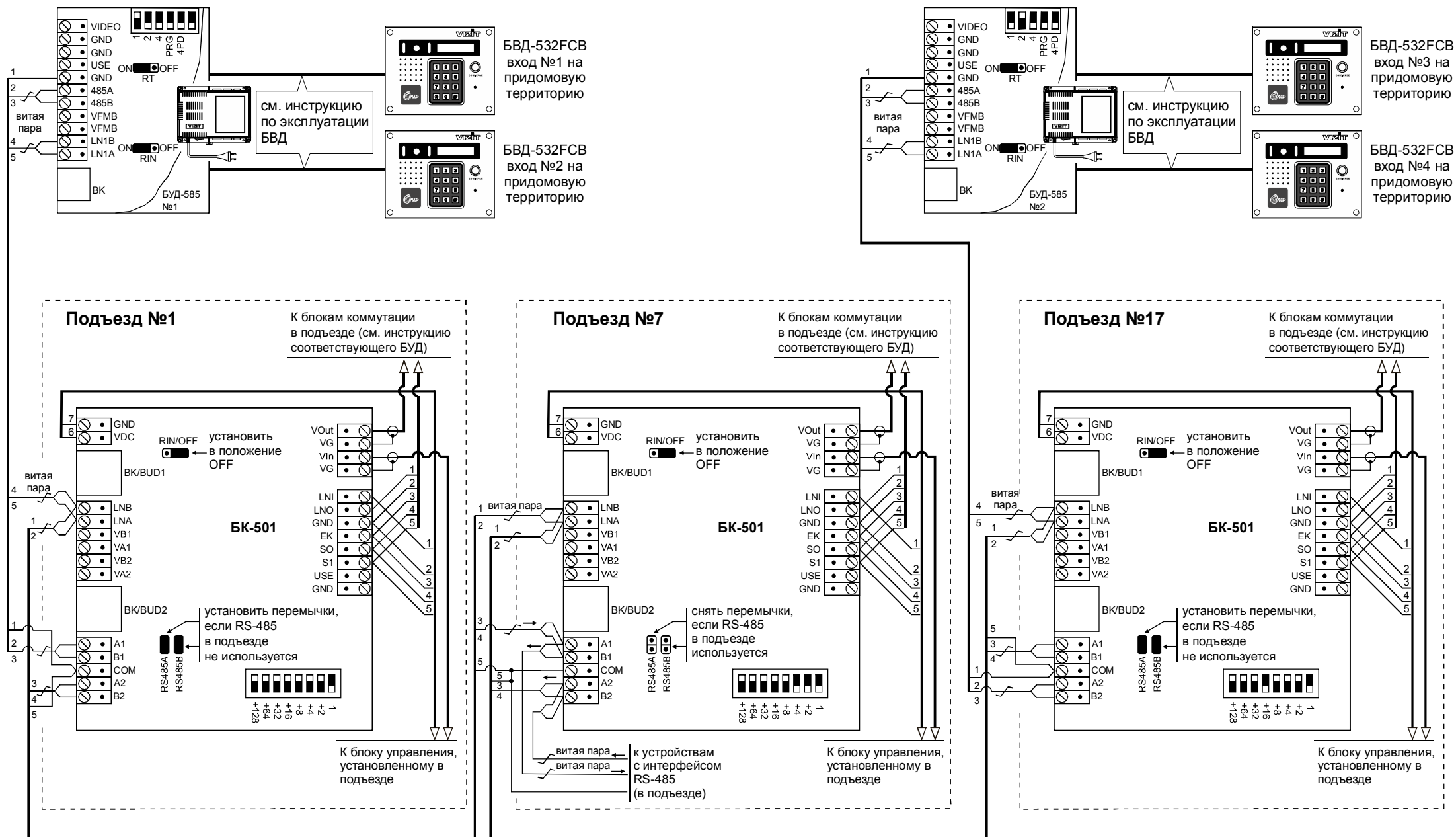
Рисунок 9 - Пример клеммного соединения блоков управления БУД-585 с блоками коммутации БК-501, установленными
