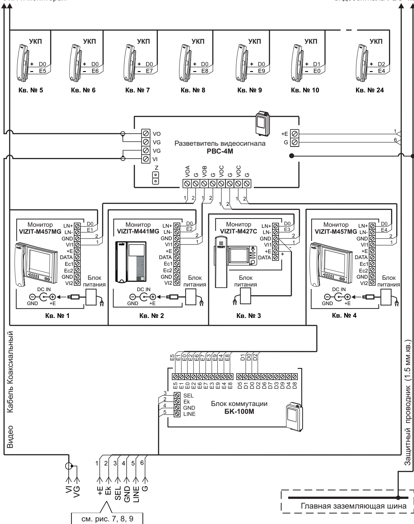
Рисунок 17 - Схема соединений блока вызова БВД-306СР-6 ( БВД-306ФСР-6 ) с блоком коммутации БК-100М , разветвителями видеосигнала PBC-4M и мониторами VIZIT в составе многоабонентского видеодомофона до 24 абонентов
