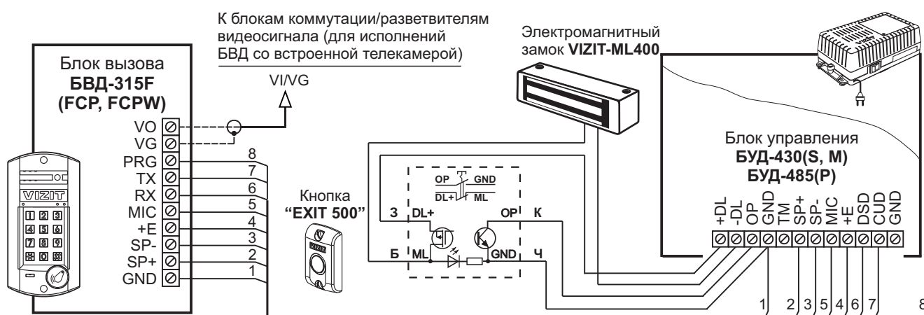
Рисунок 10 - Схема соединений блока вызова БВД-315F(FCP, FCPW) с блоком управления БУД-430(С, М), БУД-485(Р), электромагнитным замком VIZIT-ML400 и кнопкой "EXIT 500"
