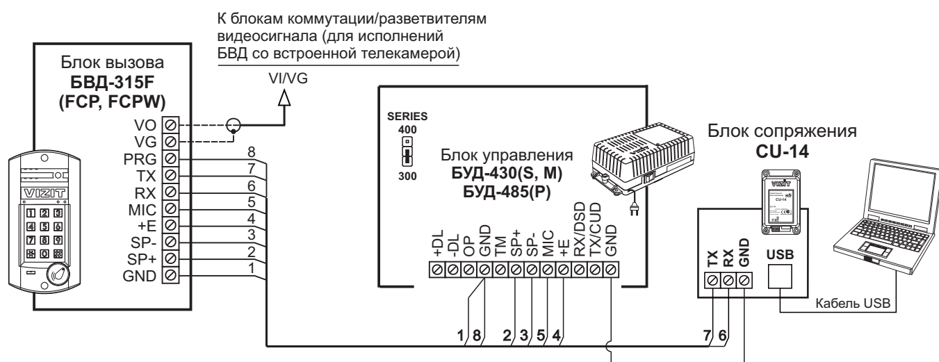
Рисунок 13 - Схема соединений блока вызова с блоками управления БУД-430(С, М) , БУД-485(Р) и блоком сопряжения CU-14
