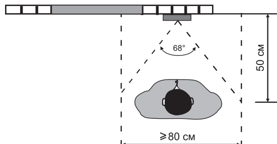
Рисунок 4 - Рекомендуемая высота установки блока вызова и область обзора телекамеры
