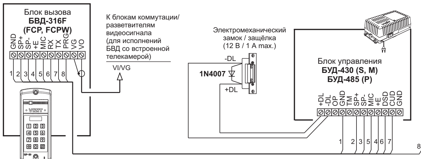
Рисунок 10 - Схема соединений блока вызова БВД-316F(FCP, FCPW) с блоками управления БУД-430 (S, М), БУД-485 (Р) , электромагнитным замком VIZIT-ML400 и кнопкой EXIT 500
