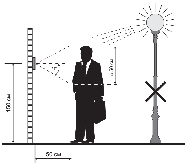
Рисунок 4 - Рекомендуемая высота установки блока вызова и область обзора телекамеры
