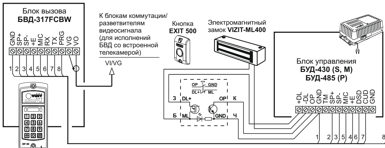
Рисунок 10 - Схема соединений блока вызова БВД-317FCBW с блоками управления БУД-430 (S, М), БУД-485 (Р) , электромагнитным замком VIZIT-ML400 и кнопкой EXIT 500
