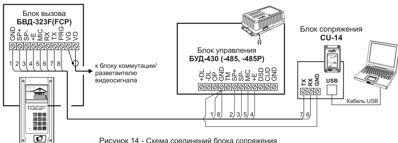
Рисунок 14 - Схема соединений блока сопряжения с блоками управления БУД-430 (-485, -485P)
