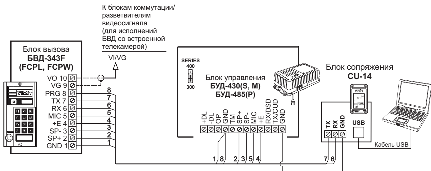
Рисунок 13 - Схема соединений блока вызова с блоками управления БУД-430(S, М), БУД-485(Р) и блоком сопряжения CU-14
