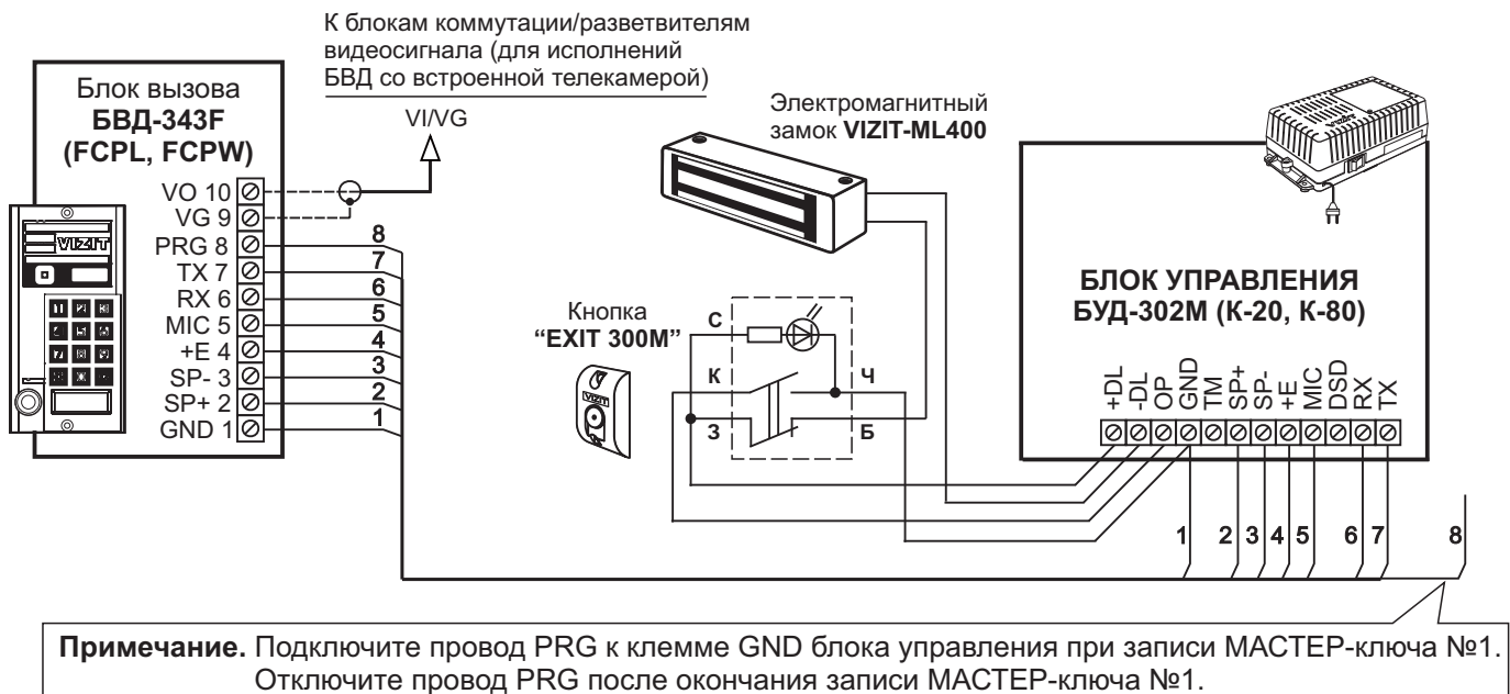
Рисунок 6 - Схема соединений блока вызова БВД-343F(FCPL, FCPW) с блоком управления БУД-302М (К-20, К-80) , электромагнитным замком VIZIT-ML400 и кнопкой “EXIT 300M”
