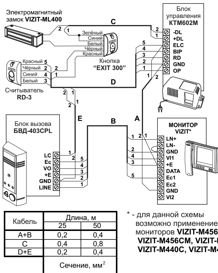
Рисунок 10 - Схема соединений БВД-403CPL с блоком управления KTM602M , считывателем RD-3 , монитором VIZIT , электромагнитным замком VIZIT-ML400 и кнопкой “EXIT 300”
