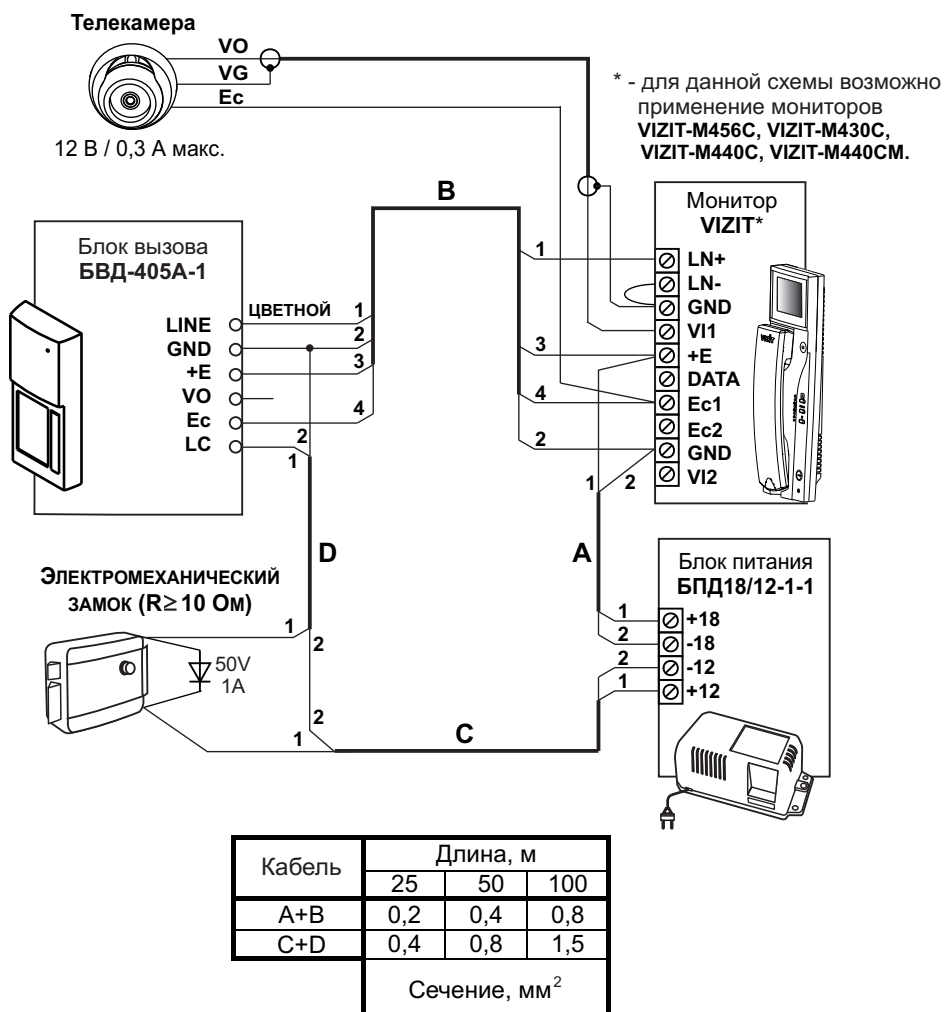
Рисунок 8 - Схема соединений БВД-405А-1 с внешней телекамерой, монитором, блоком питания БПД18/12-1-1
