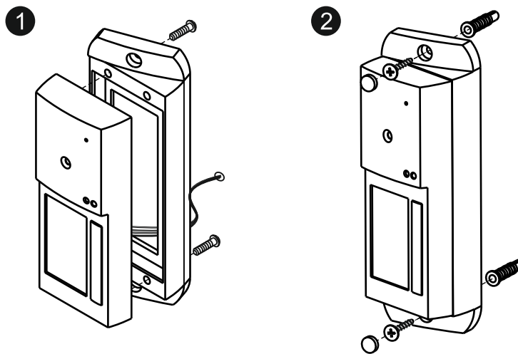
Рисунок 3 - Установка блока справа от двери
