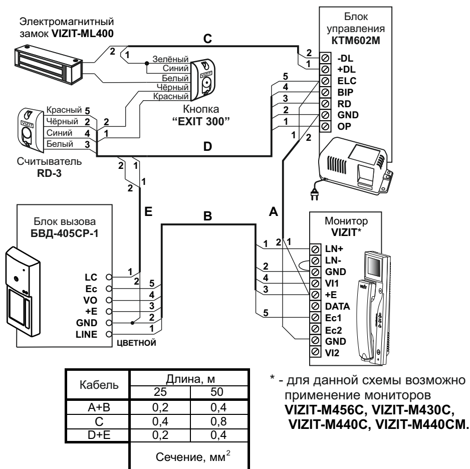
Рисунок 10 - Схема соединений БВД-405СР-1 с блоком управления КТМ602М, считывателем RD-3, монитором, электромеханическим замком VIZIT-ML400 и кнопкой "EXIT 300"
