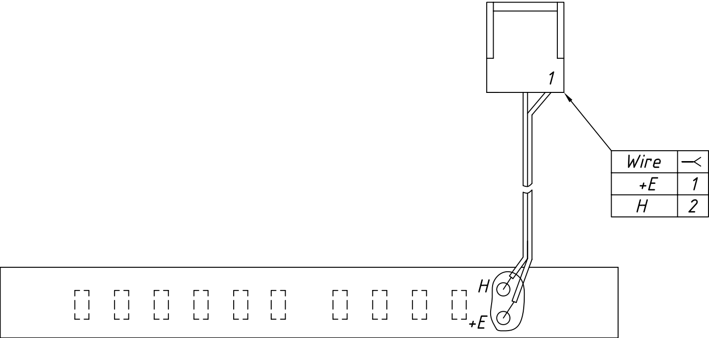
Плата подогрева Сборочный чертеж
