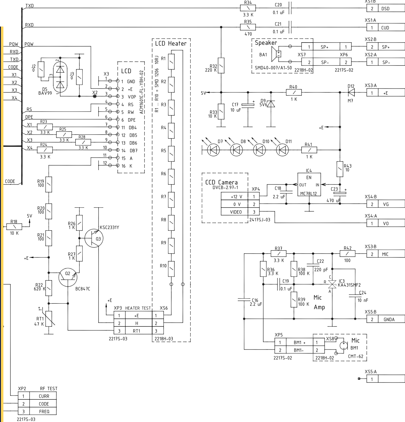
Блок вызова БВД-432 RCB Схема электрическая принципиальная
