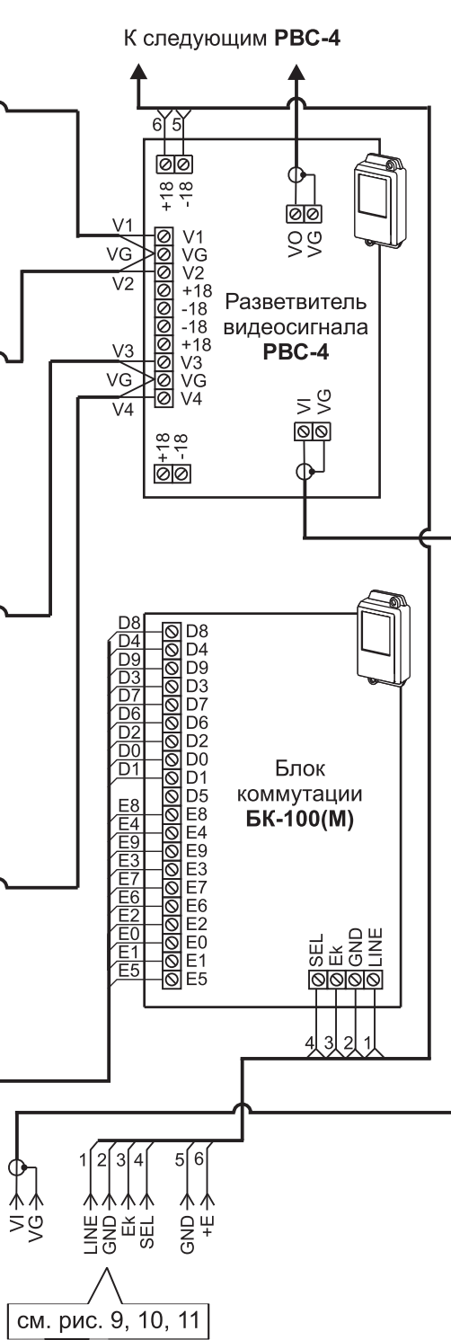
Рисунок 21 - Схема соединений блока вызова БВД-SM101RCPL(TCPL) с блоками коммутации БК-100(М) , разветвителями видеосигнала РВС-4 , мониторами и УКП в составе видеодомофона
