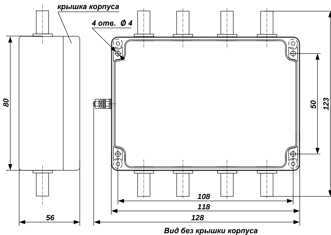
Рис. 6 Габаритные и присоединительные размеры БЗВВ-04
