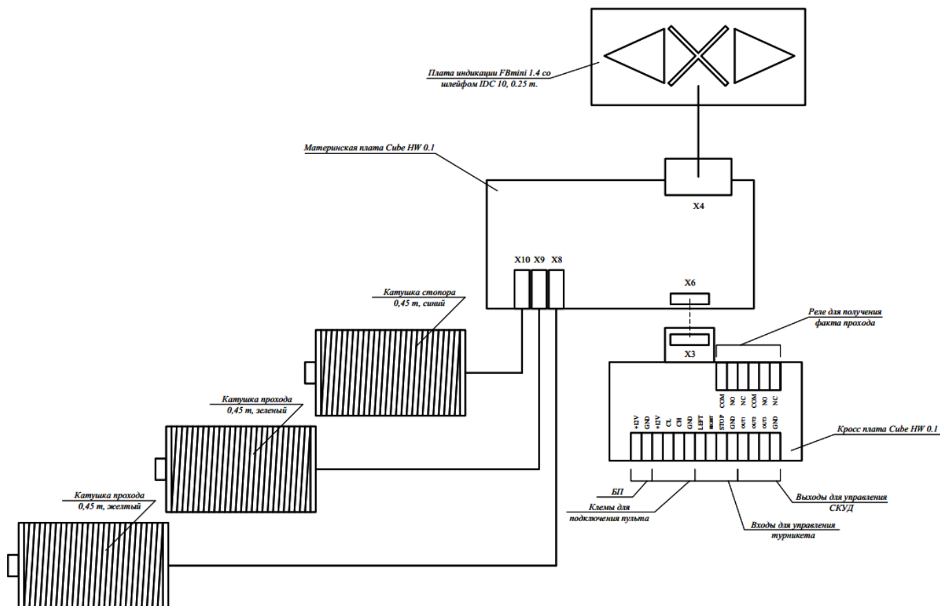
Рисунок 15 – Схема турникета
