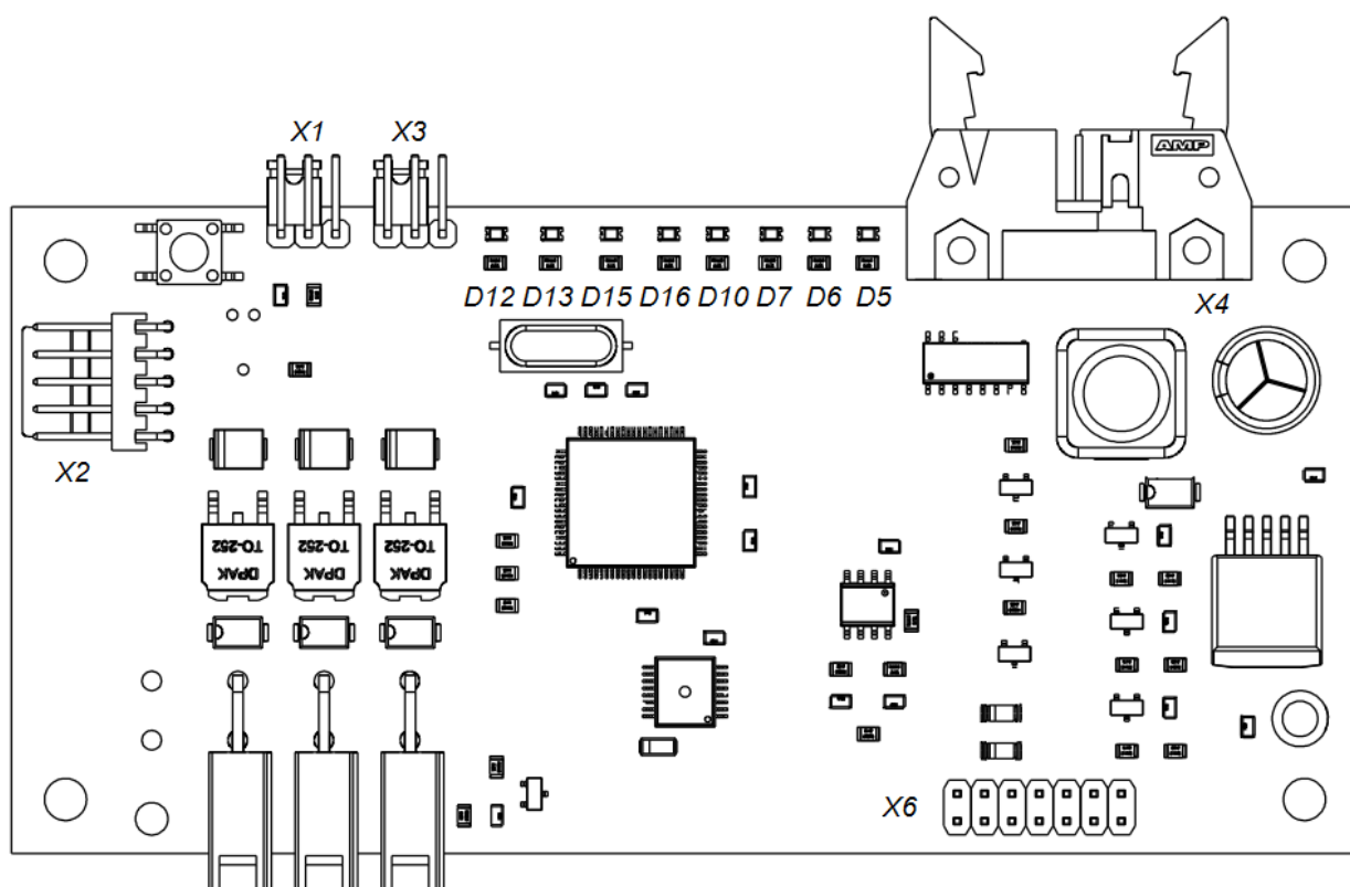
Рисунок 9 – Внешний вид материнской платы
