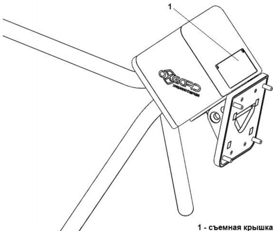
Рисунок 6 – Расположение кросс-платы под съемной крышкой
