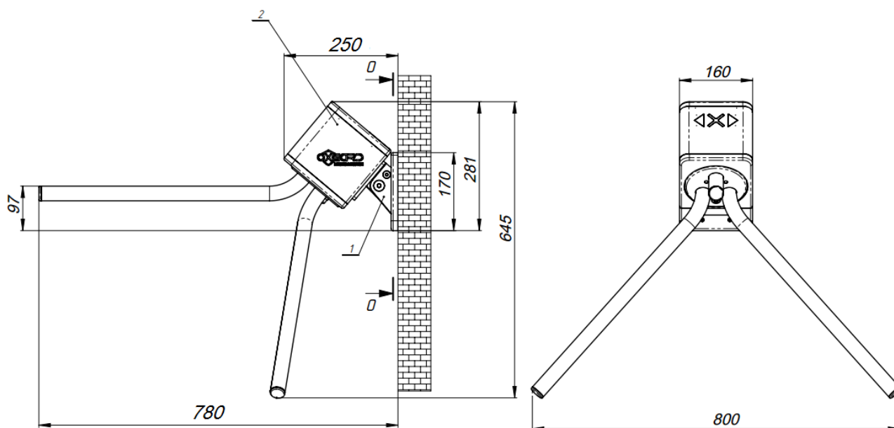
Рисунок 1 – Габаритные размеры турникета
