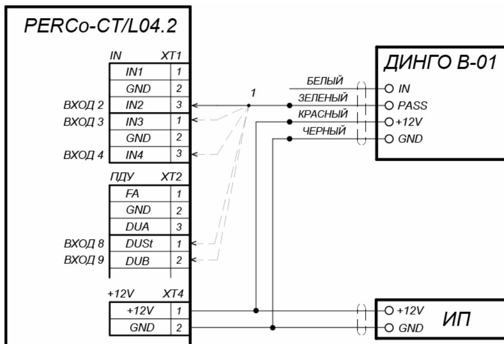
Рисунок 20. Схема подключения алкотестера «Динго В-01» (ООО СИМС-2)
