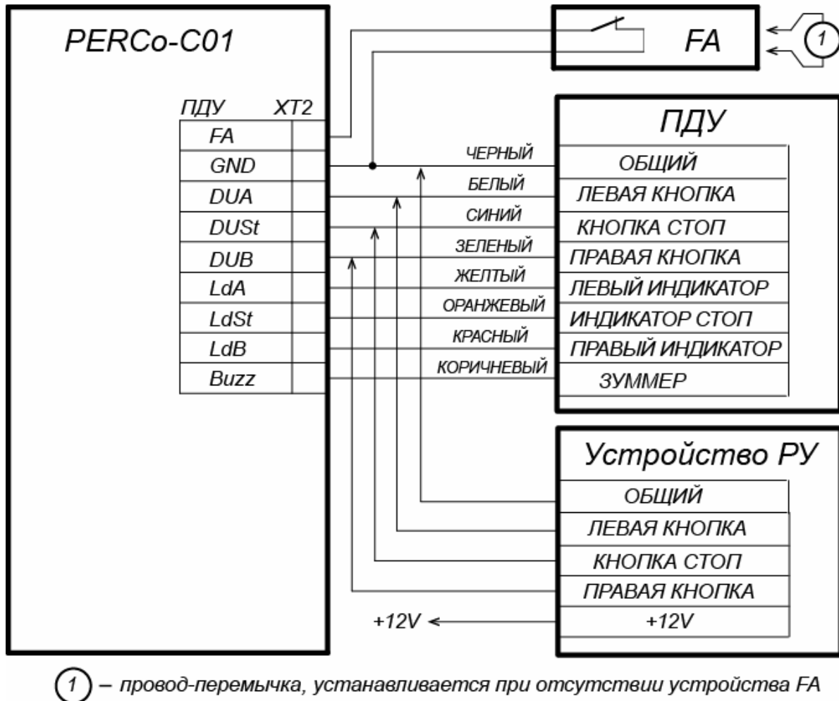
Рисунок 13. Схема подключения ПДУ или устройства РУ для варианта конфигурации «Контроллер для управления турникетом»
