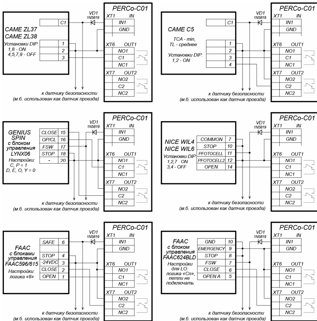
Рисунок 11. Примеры схем подключения шлагбаумов к контроллеру
