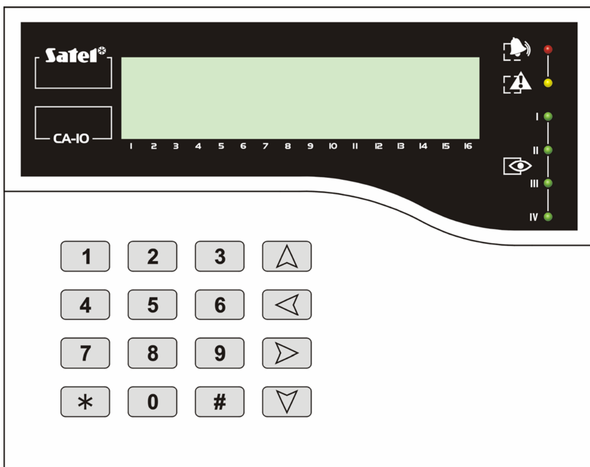
Рис. 1. Вид клавиатуры.
