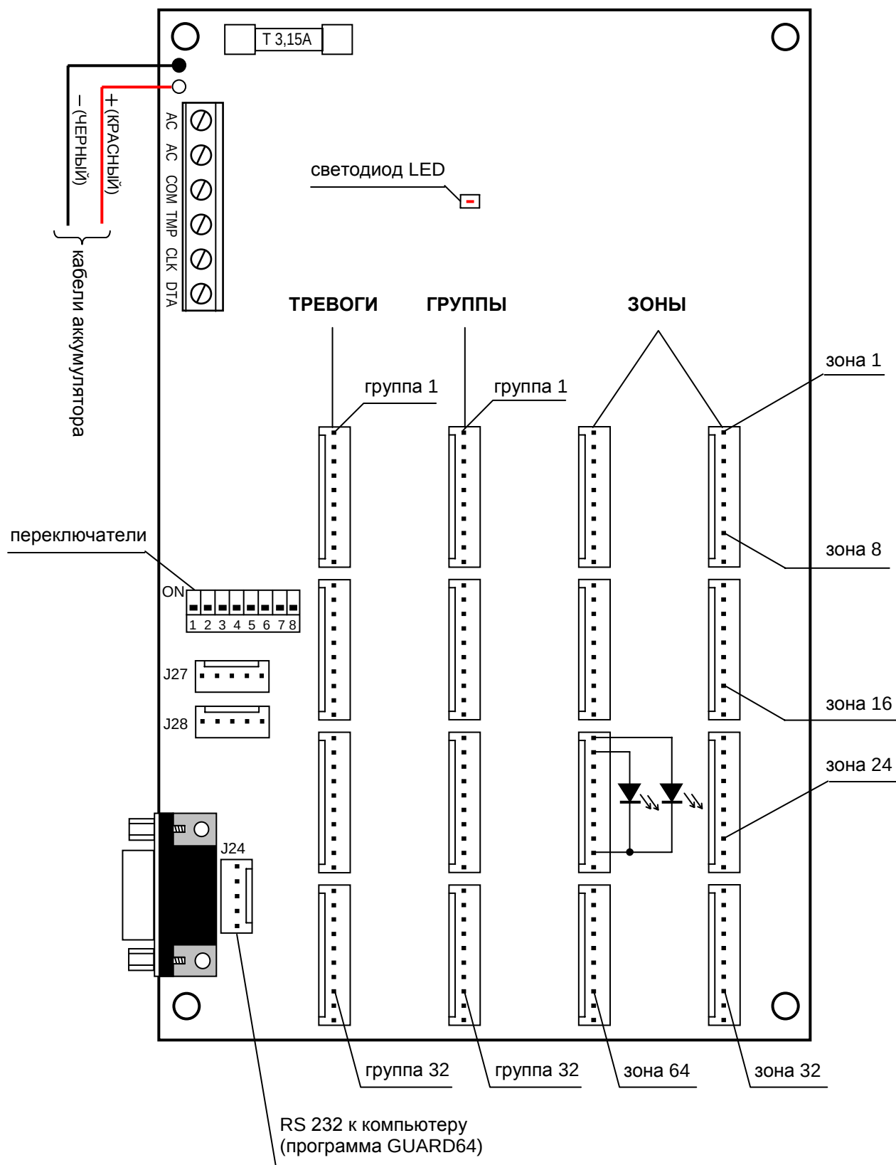
Рисунок 4. Описания контактов на плате панели индикации в случае совместной работы с ПКП СА-64.
