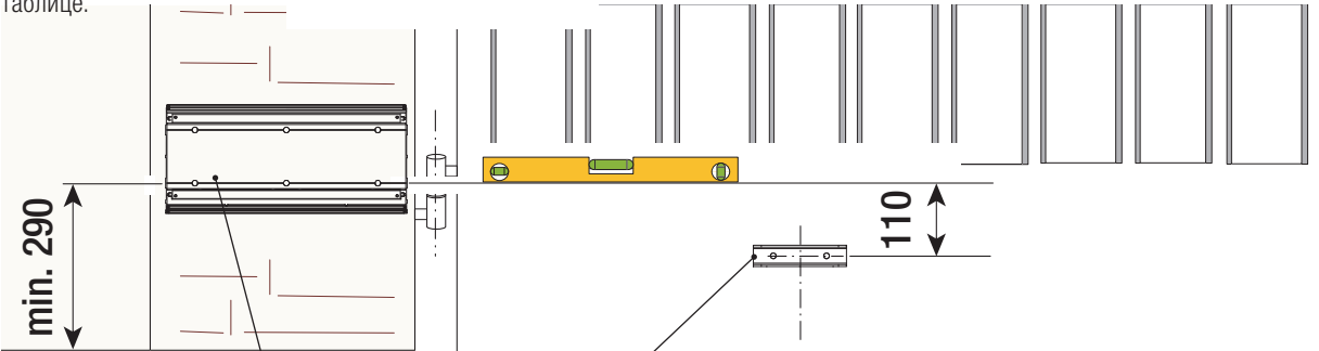
Задний кронштейн
