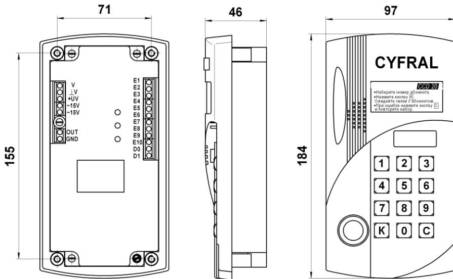
Рисунок А.2 Габаритные и установочные размеры блоков вызовЦИФРАЛ CCD-20/ТС, ЦИФРАЛ CCD-20/ТСV, ЦИФРАЛ CCD-20/ТСVC ЦИФРАЛ CCD-20/Р, ЦИФРАЛ CCD-20/PV, ЦИФРАЛ CCD-20/PVC
