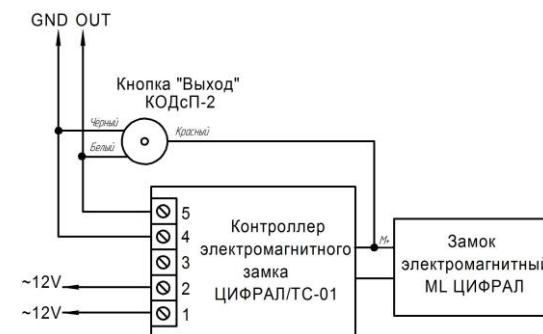
Рис. 4. Схема подключения контроллера замка ЦИФРАЛ/ТС-01 к домофону ЦИФРАЛ
