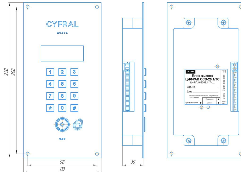
Рис. 1 Габаритные размеры блока вызова CCD-20.1/ТС (CCD-20.1/Р)
