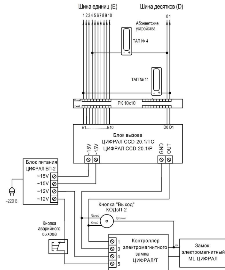
Рис. 3. Схема подключения домофона ЦИФРАЛ CCD-20.1/ТС, ЦИФРАЛ CCD-20.1/Р
