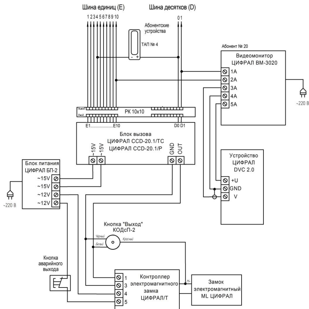
Рис.5 Схема подключения домофона ЦИФРАЛ CCD-20.1/ТС, ЦИФРАЛ CCD-20.1/Р с устройством ЦИФРАЛ DVC 2.0 и видеомонитором ЦИФРАЛ ВМ-3020
