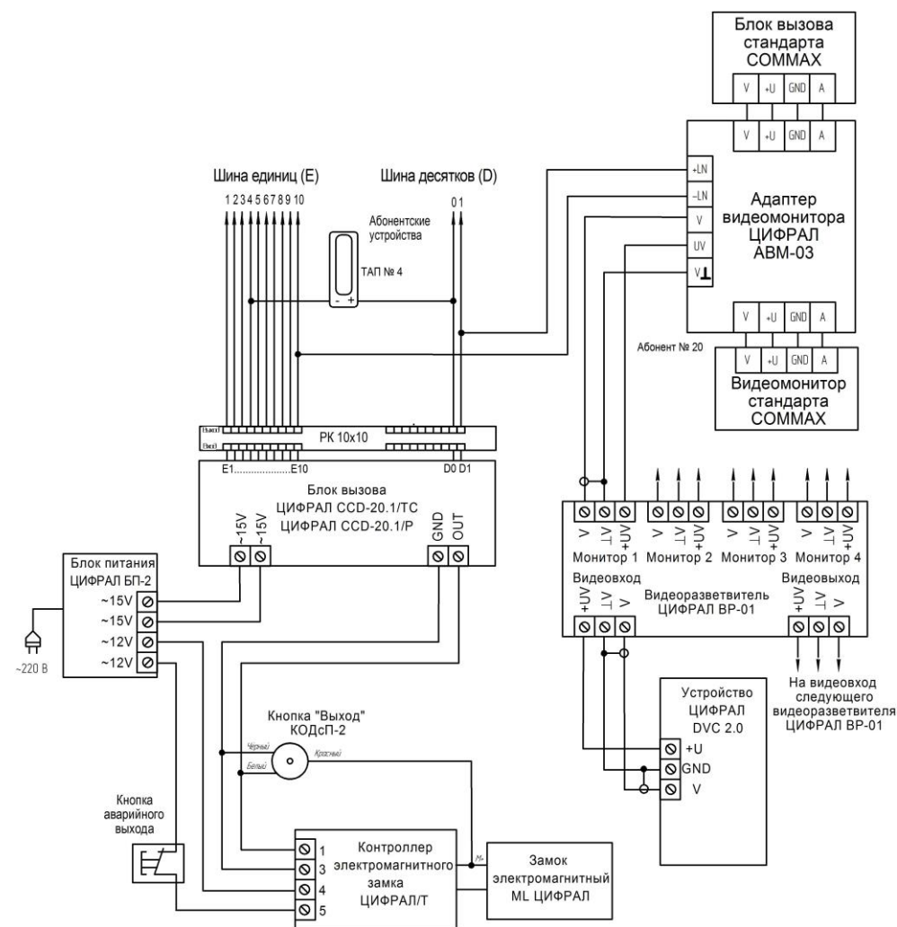
Рис.6 Схема подключения домофона ЦИФРАЛ CCD-20.1/ТС, ЦИФРАЛ CCD-20.1/Р с устройством ЦИФРАЛ DVC 2.0 и видеомонитором стандарта COMMAX (с использованием адаптера АВМ-03 и видеоразветвителями ВР-01)
