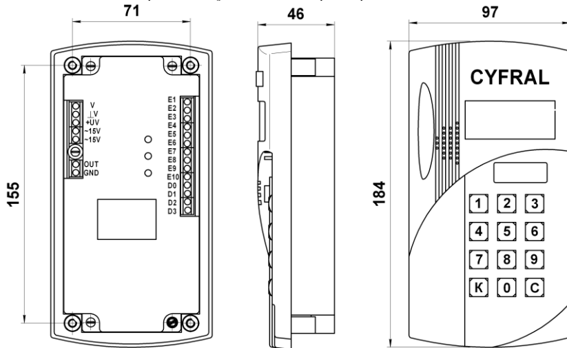
Рисунок А.1 Габаритные и установочные размеры блоков вызова ЦИФРАЛ CCD-40, ЦИФРАЛ CCD-40/V, ЦИФРАЛ CCD-40/VC
