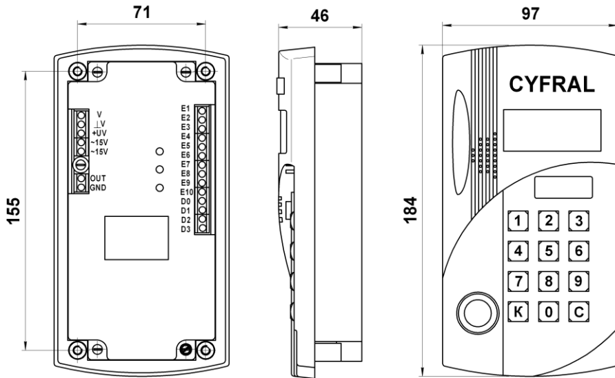
Рисунок А.2 Габаритные и установочные размеры блоков вызова ЦИФРАЛ ССД-40/ТС, ЦИФРАЛ ССД-40/ТСV, ЦИФРАЛ ССД-40/ТСVC, ЦИФРАЛ ССД-40/Р, ЦИФРАЛ ССД-40/PV, ЦИФРАЛ ССД-40/PVC
