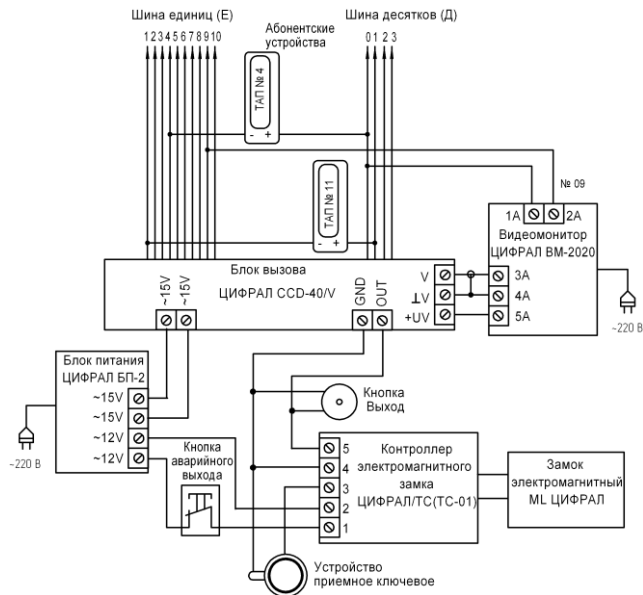
Рисунок Б.2 Схема подключения домофона ЦИФРАЛ CCD-40/V (для варианта исполнения «VC» использовать видеомонитор ЦИФРАЛ ВМ-3020)
