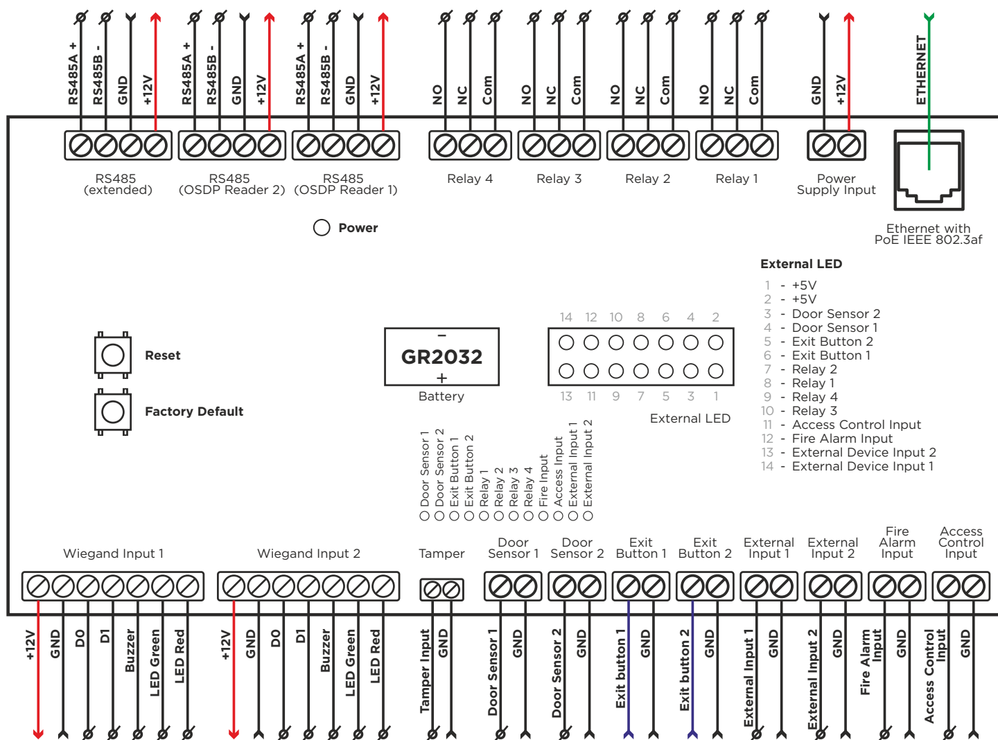
Схема подключения и назначение контактов на разъемах
