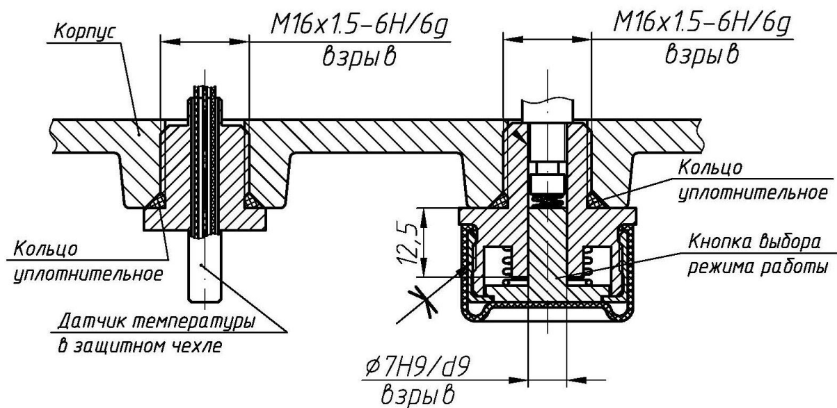
Рисунок А.4 – Датчик температуры и кнопка табло Часы-Ех – см разрез Б-Б на рис. А.1
