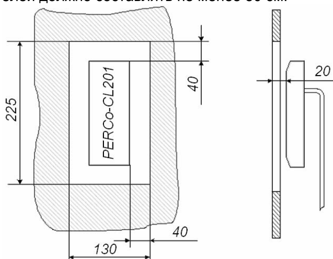
Рисунок 2. Установка контроллера за металлической поверхностью
