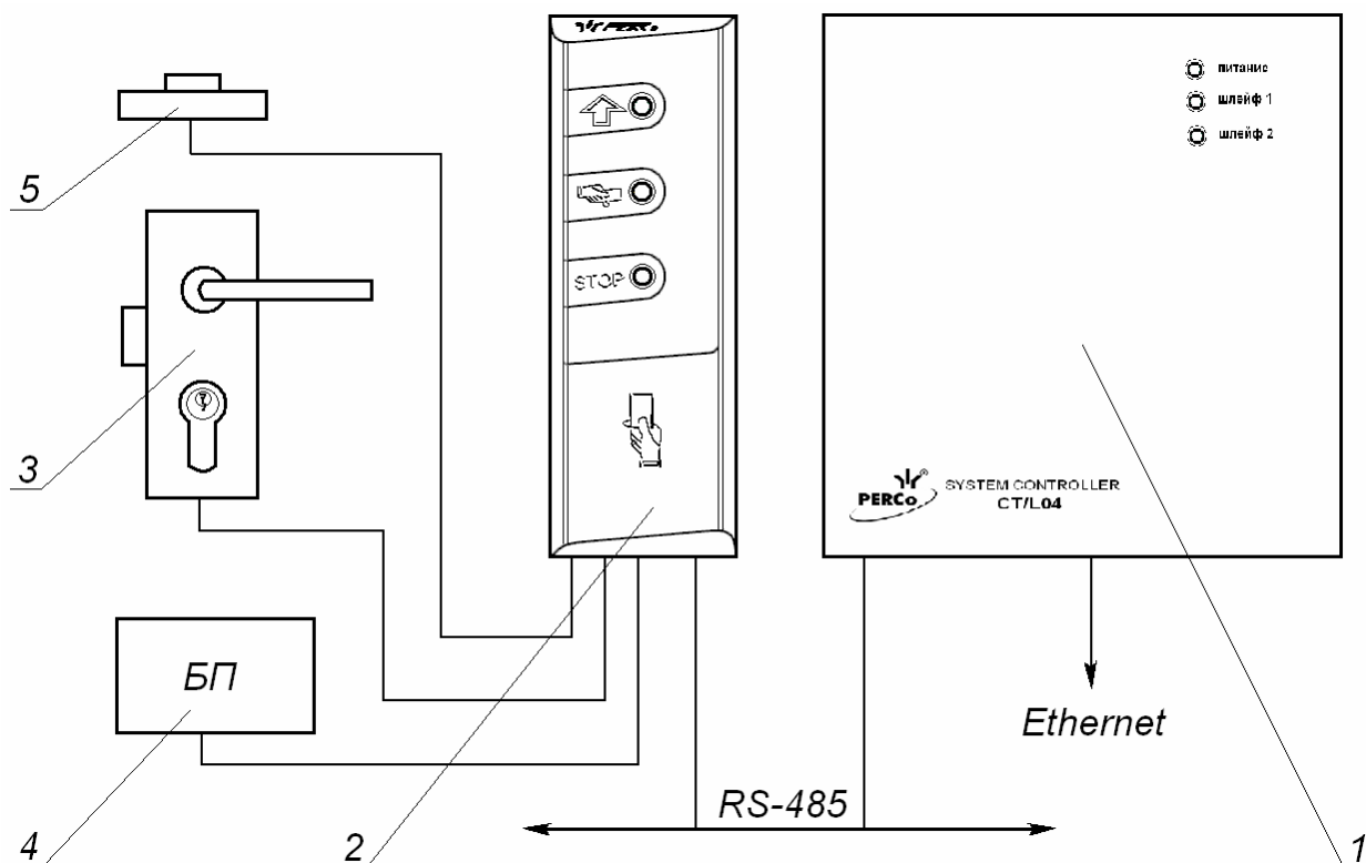
Рисунок 1. Функциональная схема
