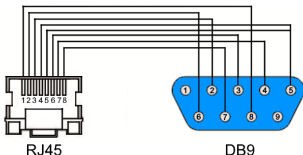
Рис.2 Распиновка разъемов кабеля Console-RJ45-DB9F
