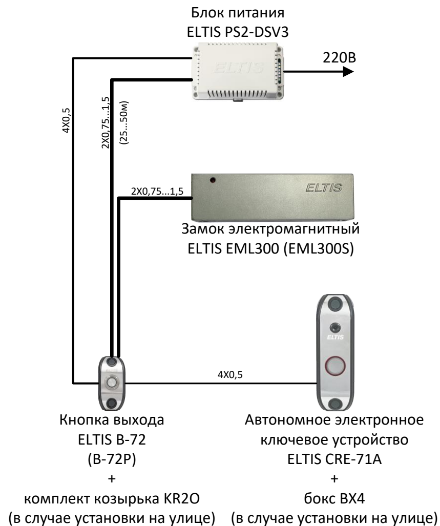
Вариант 2: С использованием функции аварийного открывания двери в кнопке выхода
