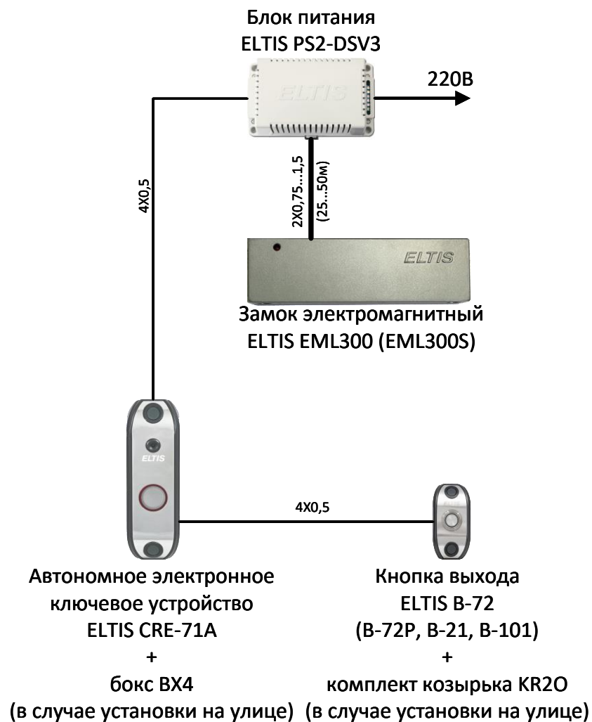
Вариант 1: Без использования функций аварийного открывания двери в кнопке выхода
