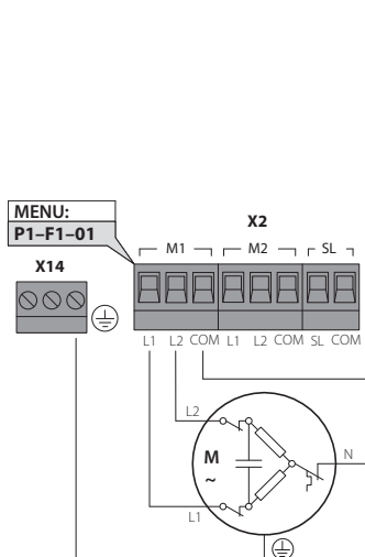
Рисунок 2. Подключение привода одностворчатых ворот
