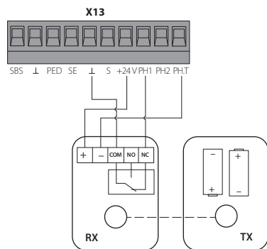
Рисунок 7. Подключение фотоэлементов с батареями, срабатывающих при закрывании
