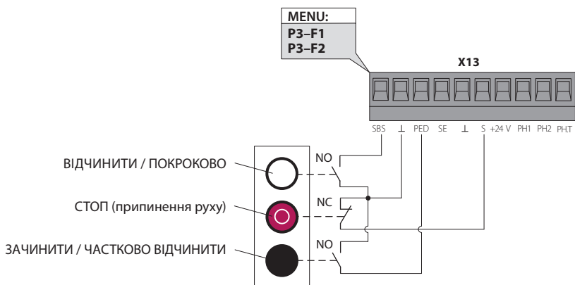
Рисунок 4. Підключення кнопочного поста керування
