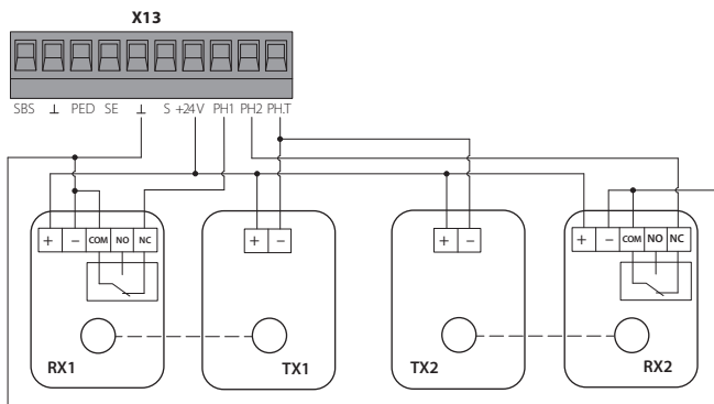
Рисунок 6. Подключение фотоэлементов, срабатывающих при закрывании и открывании
