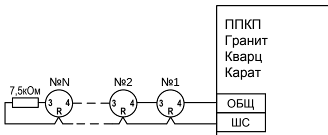
Рис.3 Схема подключения извещателей к ППКП «Гранит», «Кварц» и «Карат» производства ООО НПО «Сибирский Арсенал».
