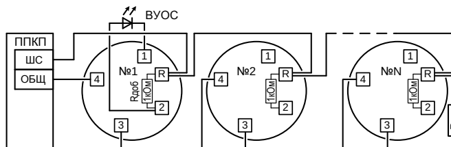
Рис.1 Типовая схема подключения извещателей к ППКП со знакопостоянным ШС. Величина оконечного резистора Rок определяется в соответствии с техническим описанием ППКП. Добавочный резистор Rдоб по умолчанию установлен – 1 кОм.
