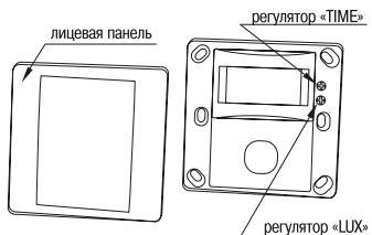
Рисунок 12 – Конструкция датчика движения ДД-029
