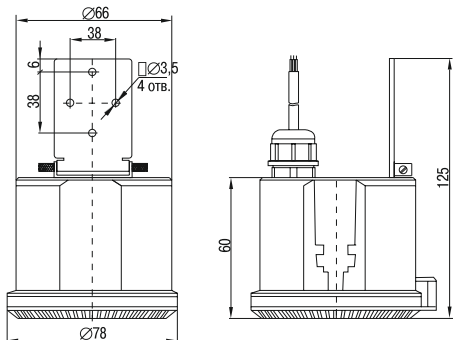
Рисунок 9 – ДД-МВ601
