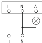
Рисунок 12 – Схема подключения датчика ДД-МВ301
