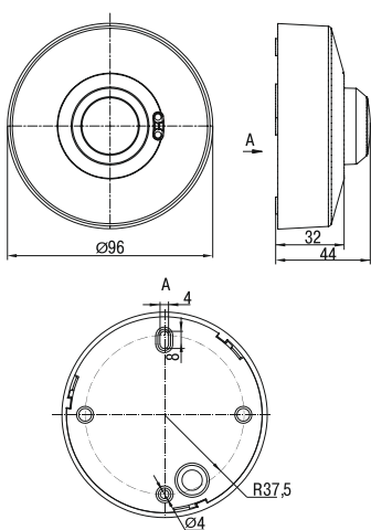
Рисунок 4 – ДД-МВ101
