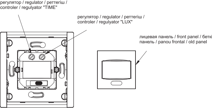
Рисунок 3 – Конструкция датчика / Figure 3 – Sensor design / 3 сурет – Датчигінің құрылымы / Figura 3 – Designul senzorului / 3-rasm – Sensorining konstruksiyasi
