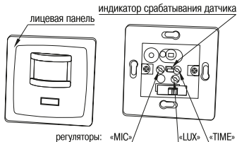
Рисунок 15 – Конструкция датчика движения ДД-035
